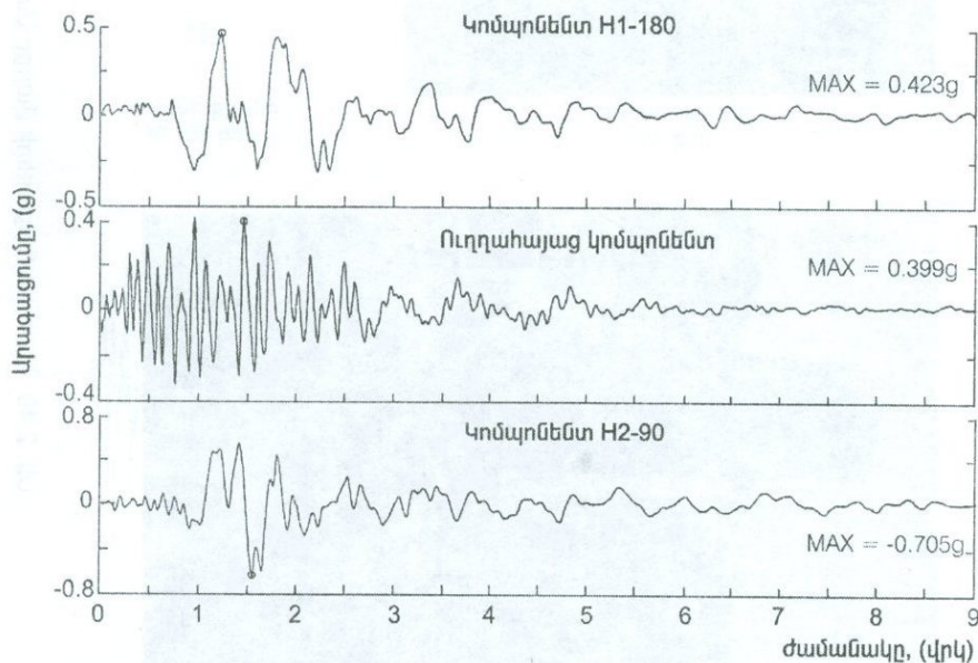
Նկ. 2.42 CIG կայանում գրանցված երկրաշարժի աքսելերոգրամը [85] (Սան-Մալվադոր, 10 հոկտեմբեր, 1986):
