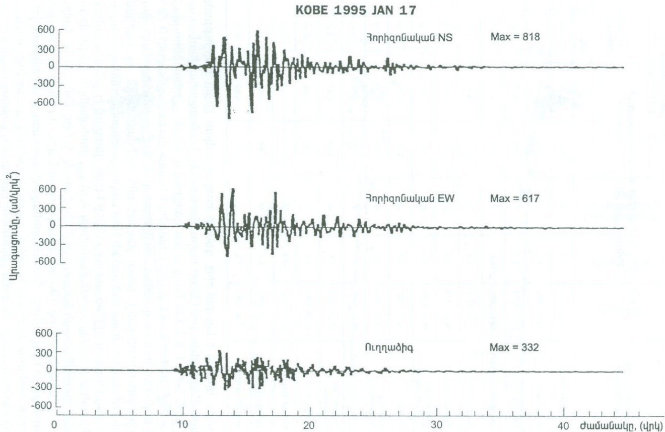
Նկ. 2.28.13 1995թ. հունվարի 17-ի Կոբեի երկրաշարժի արժեքները [147]:
