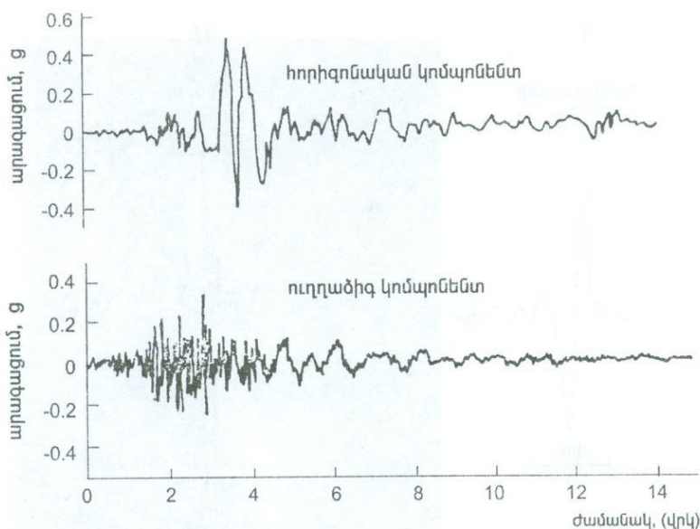
Նկ. 2.38 Պարկֆիլդի 1966թ. հունիսի 27-ի երկրաշարժի աքսելերոգրամը [40]:
