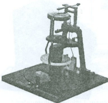
դ. Վիլնոտի սեյսմոսկոպ
