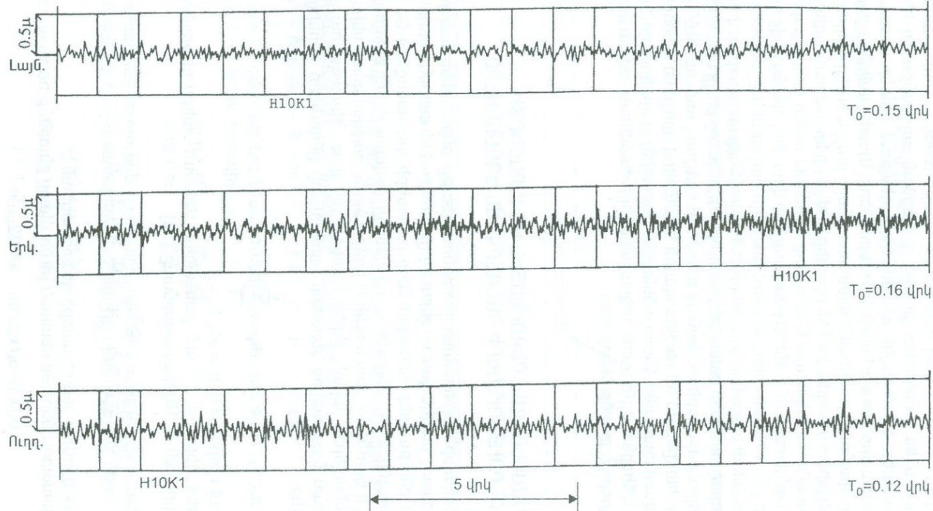
Նկ. 2.13 Հայսեյսմիկ զճի (Երևան) տարածքում գրունտի միկրոտատանումների եռակոմպոնենտ գրանցումները
