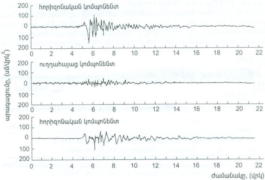
Նկ. 3.16 Սպիտակի երկրաշարժի ժամանակ Ղուկասյանում (Աշոցք) գրանցված գետնի աքսելերոգրամները հիմնական հարվածի և առաջին հետհարվածի ընթացքում:
