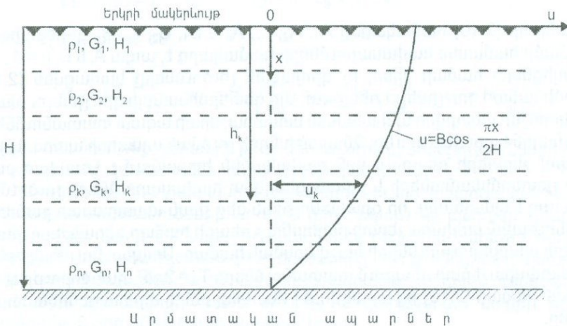
Նկ. 2.14 Անհամասեռ գործնտային ստվարաշերտի հաշվարկային սխեման
