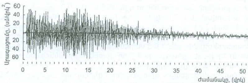
Նկ. 2.16 1988թ. դեկտեմբերի 7 - ի Սպիտակի երկրաշարժի Երևանում գրանցված աքսելերոգրամը (ԻՍԶԿ N3 բազալտներ Երևան, Ա. Ավետիսյան փ.1) [60]:
