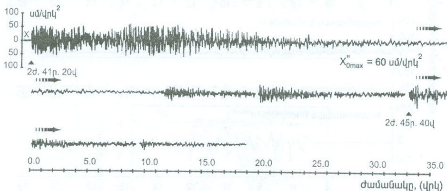
Նկ. 3.17 Սպիտակի երկրաշարժի ժամանակ Երևանում գրանցված գետնի աքսելերոգրամ հիմնական և հետագա հետհարվածների ժամանակ [60]:
