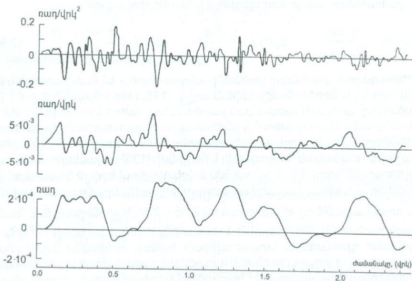
Նկ. 2.35 Գրունտի պտտական շարժումների կինեմատիկական պարամետրերը, ստացված Զերցեգնովի կայանում գրանցված գրունտի հորիզոնական կոմպոնենտների շարժումներից (սկզբնական ուժեղ ցնցումների փուլում [52]):
