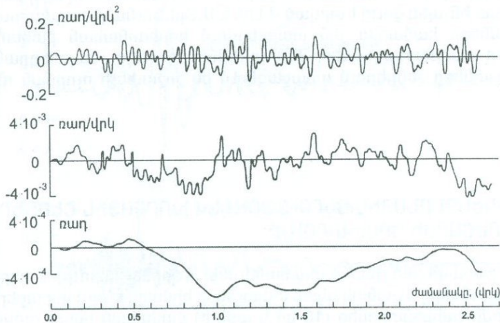
Նկ. 2.36 Գրունտի պտտական շարժումների կինեմատիկական պարամետրերը, ստացված Ուլցինժի կայանում գրանցված գրունտի հորիզոնական կոմպոնենտների շարժումներից (սկսնական ուժեղ ցնցումների փուլում [52]):
