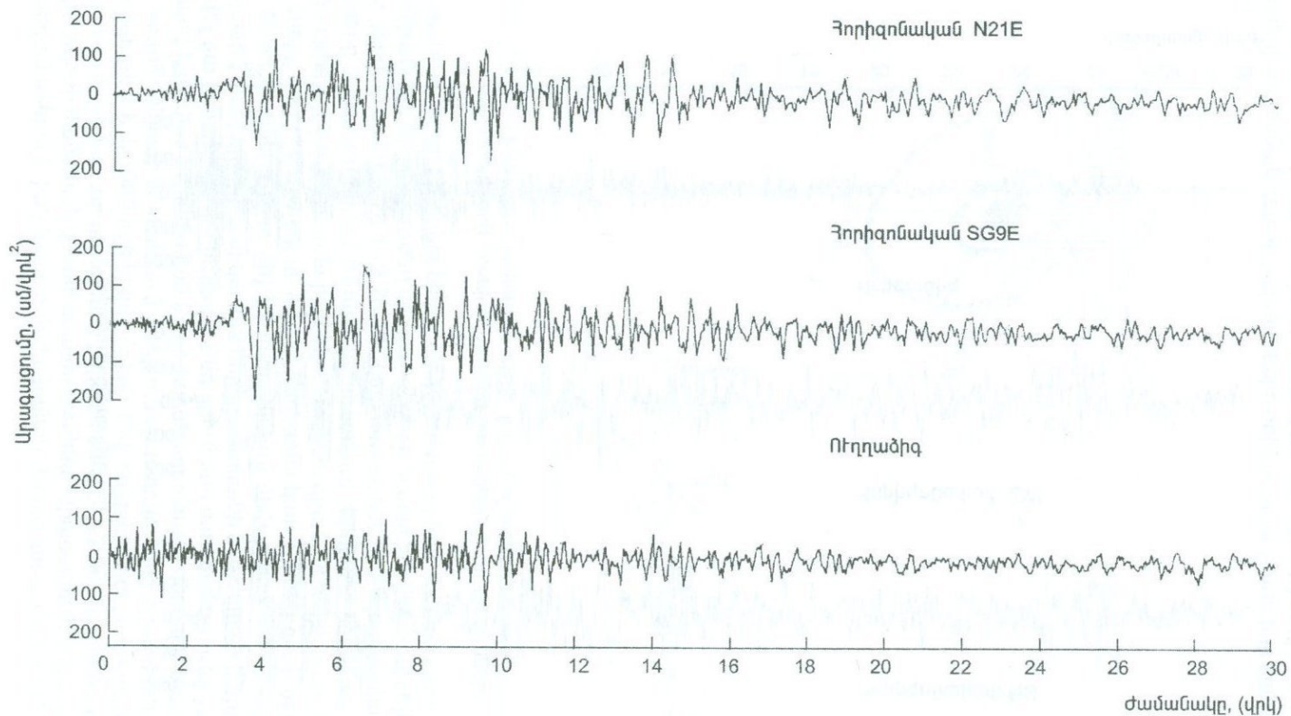
Նկ. 2.28.2 1952թ.-ի հուլիսի 21-ի Թաֆտի երկրաշարժի եռակոմպոնենտ աքսելերոգրամները [137]:
