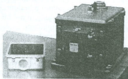
դ. CCP3 (երեք կոմպոնենտ) T_w = 0.05 վրկ, h = 0.6 (НФЗ Москва)
