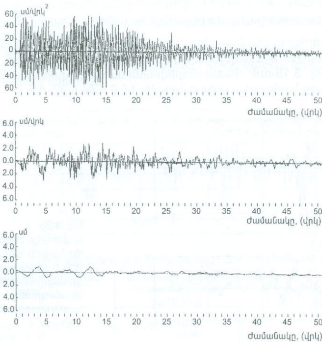
Նկ. 3.18 Սպիտակի երկրաշարժի ժամանակ Երևանում գրանցված գետնի աքսելերոգրամը և նրանից ինտեգրման միջոցով ստացված վելիստոգրամը և սեյսմոգրամը:
