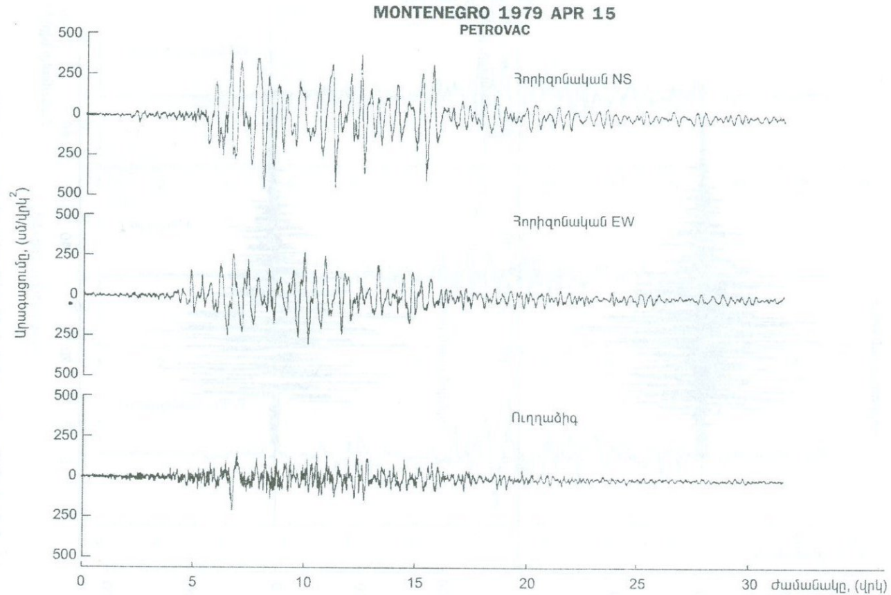
Նկ. 2.28.7 1979թ. ապրիլի 15-ի Մոնտենեգրոյի երկրաշարժերի արբւելերոգրամները [129,139]:
