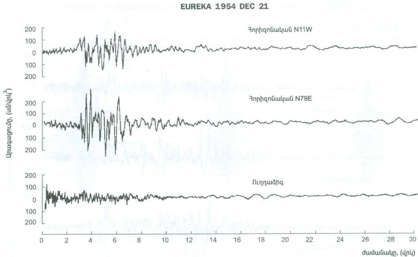
Նկ. 2.28.3 1954թ. դեկտեմբերի 21-ի Յուրկայի երկրաշարժի աքսելերոգրամները [137]:
