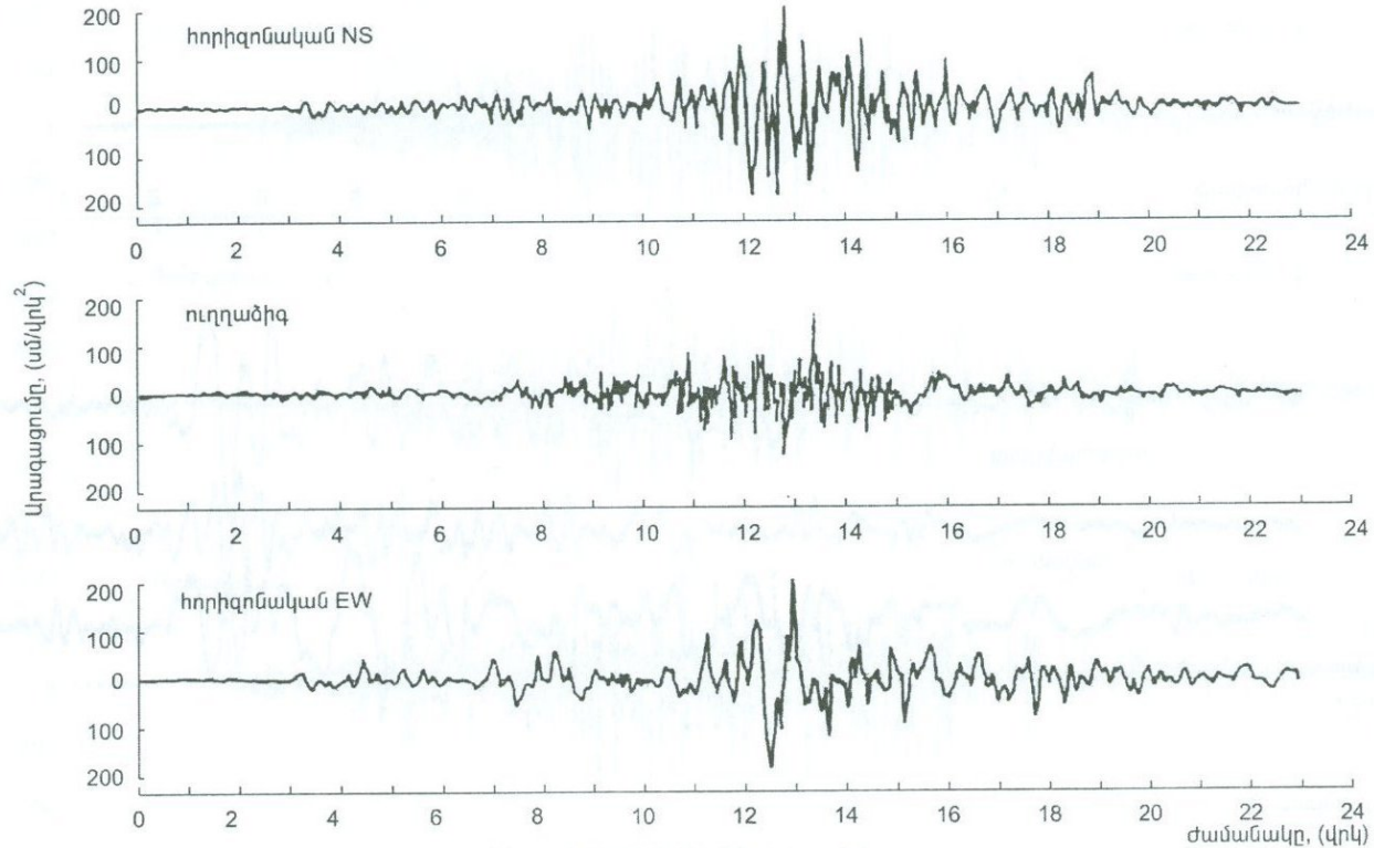
Նկ. 2.28.9 1988թ. դեկտեմբերի 7-ի Սպիտակի երկրաշարժի արժեքները [20, 86]:
