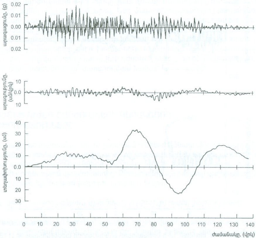
Նկ. 2.3 1964թ. հուլիսի 6-ի Մեխիկոյի երկրաշարժի աքսելերոգրամը և նրանից ստացած վեխոգրամը և սեյսմոգրամը [39]:
