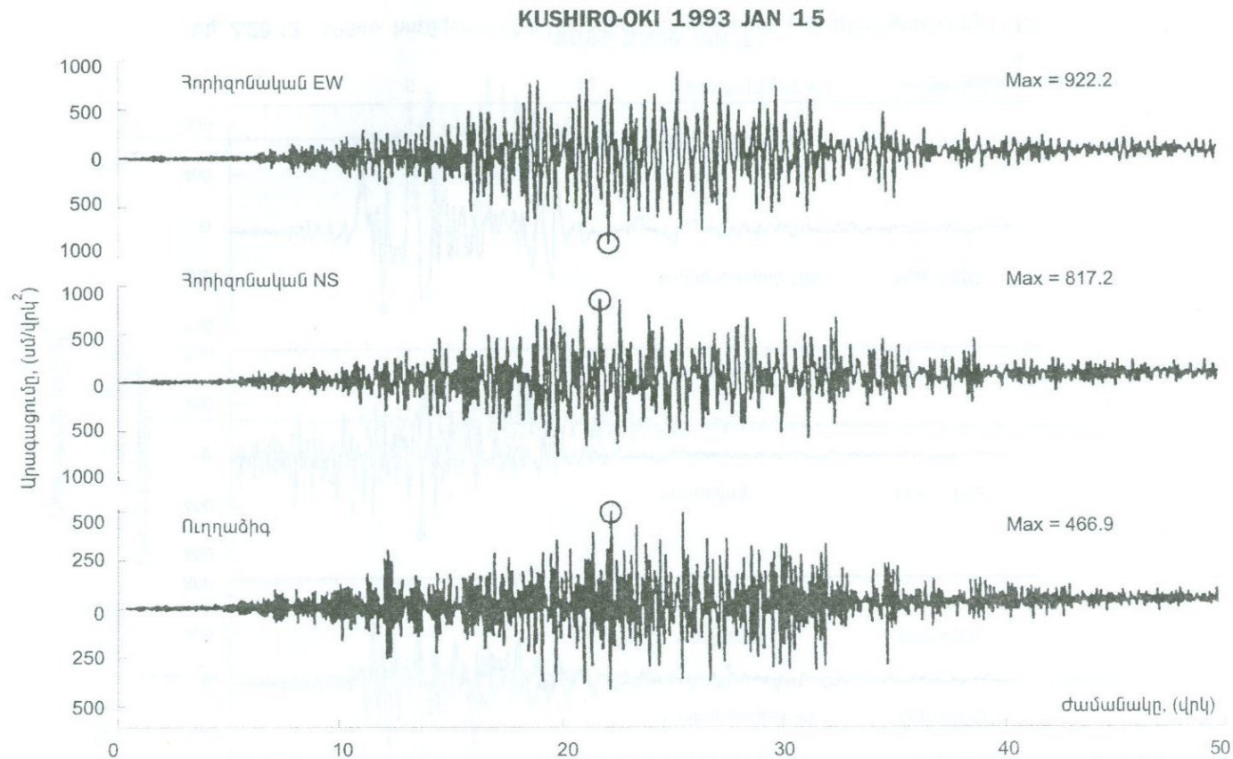
Նկ. 2.28.11 1993թ. հունվարի 15-ի Կուշիռ-Օկի երկրաշարժի արբելերոգրամները [120]:
