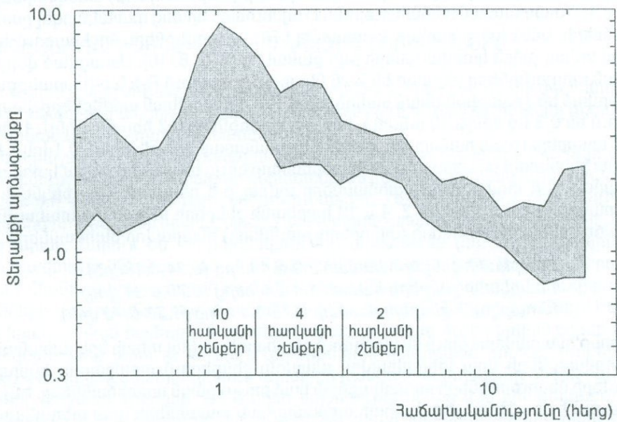
Նկ. 2.26 Սան-Ֆրանցիսկո քաղաքի տարբեր գրունտային տեղանքների արժագանքի սպեկտրները:
