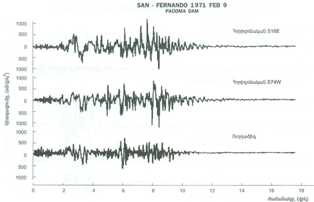
Նկ. 2.28.4 1971թ. փետրվարի 9-ի Սան-Ֆերնանդոյի երկրաշարժի աքսելերոգրամները [118]:
