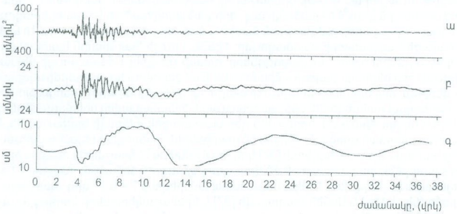
Նկ. 1.26 Ուժեղ երկրաշարժի արսելերոգրամը (ա.) և նրանից ինտեգրման եղանակով ստացած վելիտոգրամը (բ.) և սեյսմոգրամը (գ.):
