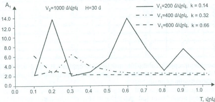
Նկ. 2.23 Երկրի մակերևույթի վրա տատանումների սաստկացումը՝ կախված ընկնող ալիքի պարբերությունների մեծություններից:
