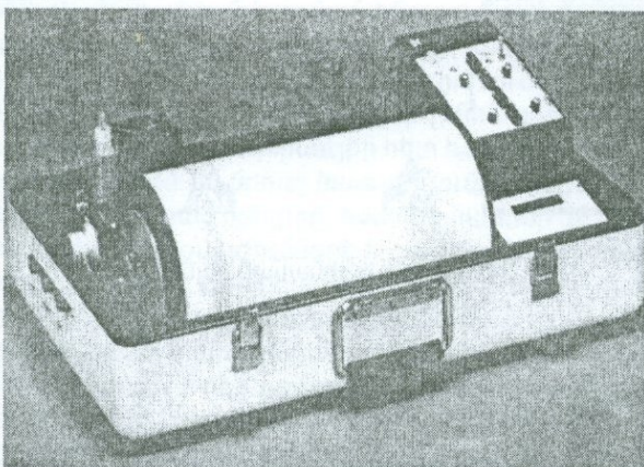
Նկ. 1.19 Ամերիկյան Kinematics PS-2 տիպի սեյսմոգրաֆի գրանցող սարքը:
