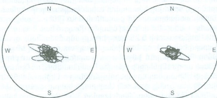
Նկ. 3.22 CBM սեյսմոսկրայի գրանցումները Լենինականում:
