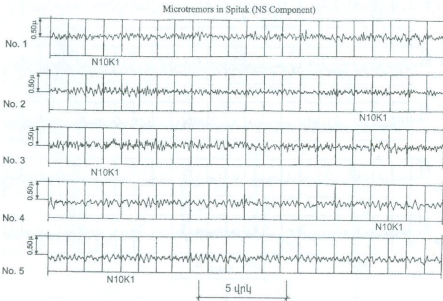
Նկ. 2.12 Սպիտակ քաղաքի տարբեր տեղամասերի միկրոտատանումների գրանցումները [114, 136, 142]:
