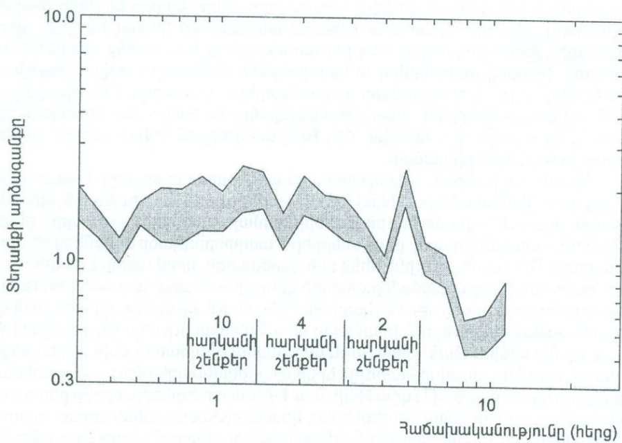
Նկ. 2.26 Սան-Ֆրանցիսկո քաղաքի տարբեր գրունտային տեղանքների արժագանքի սպեկտրները:
