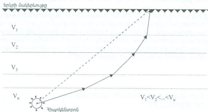
Նկ. 2.5 սեյսմիկ ալիքի տարածման ուղին:
