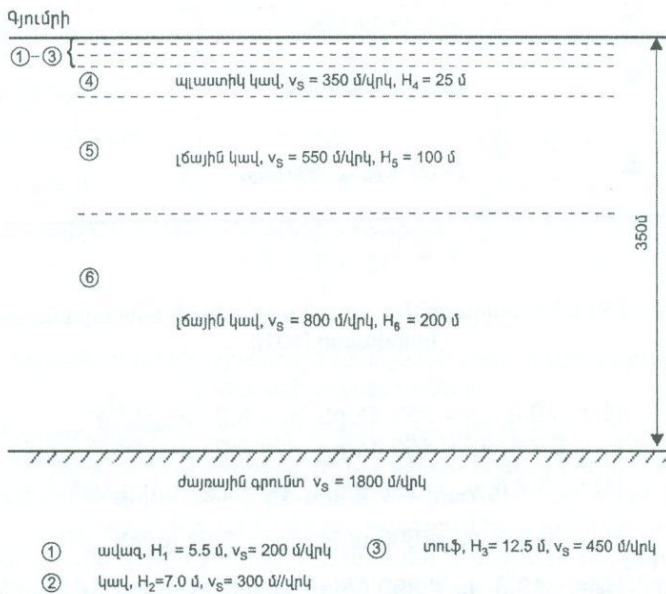
Նկ. 2.18 Գյումրի քաղաքի կենտրոնական մասի երկրաբանական կտրվածքի սխեման [97, 152]:
