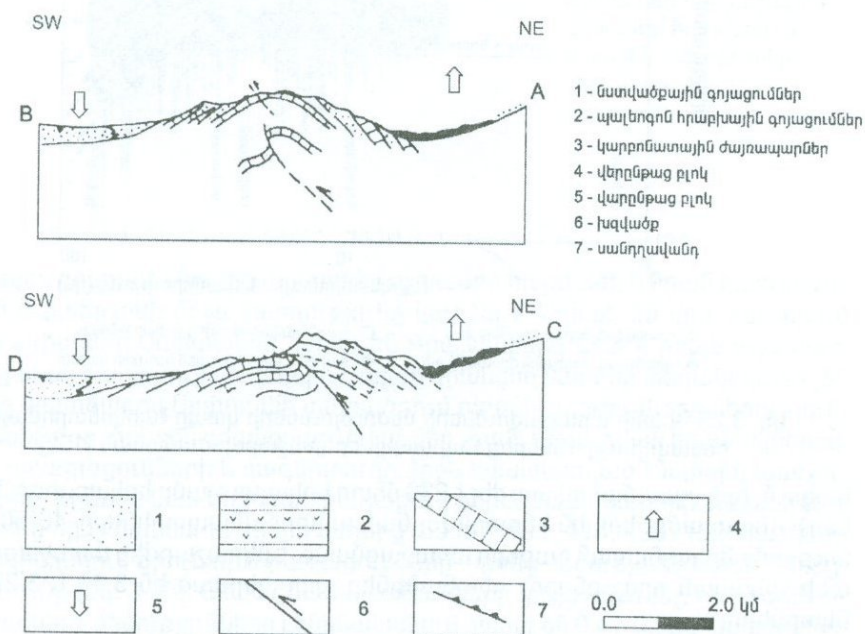
Նկ. 3.26 Սափիտակի երկրաշարժի ժամանակ առաջացած մակերևութային խզվածքի գեոմորֆոլոգիական դրությունը և խզվածքի ուղղահայաց ուղղությամբ երկրաբանական կտրվածքները [136]:
