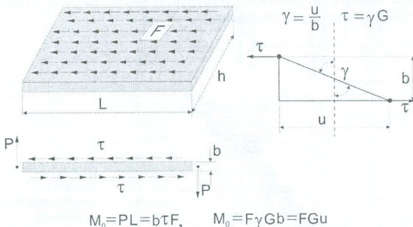
Նկ. 1.45 Տրոհման պրոցեսի մեխանիկական և երկրաշարժի M_0 մոմենտի առաջացման լուսաբանումը [49]:
