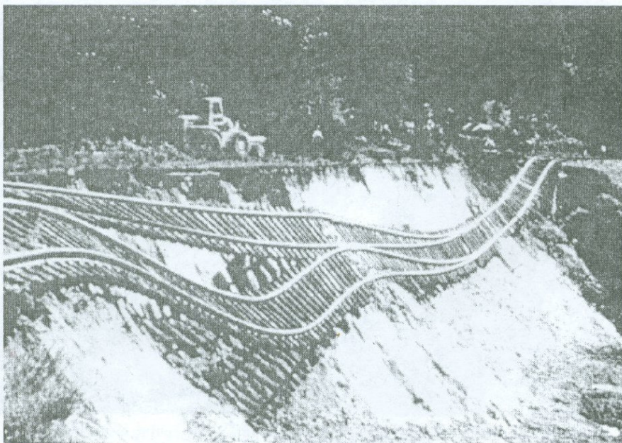
Նկ. 1.7 1965թ. Օլիմպիայի (ԱՄՆ) երկրաշարժից երկաթգծի ծոռված գծերը մնացել են օդում կախված՝ դրանց տակից բլրի հողը սողանքի հետևանքով սահել է ներքև [23, 130]:
