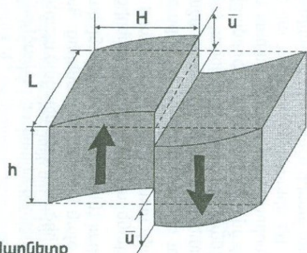
Նկ. 1.50 Միջավայրի դեֆորմացման սխեմատիկ պատկերը (a) և սահքի լարումների բաշխվածությունը:
