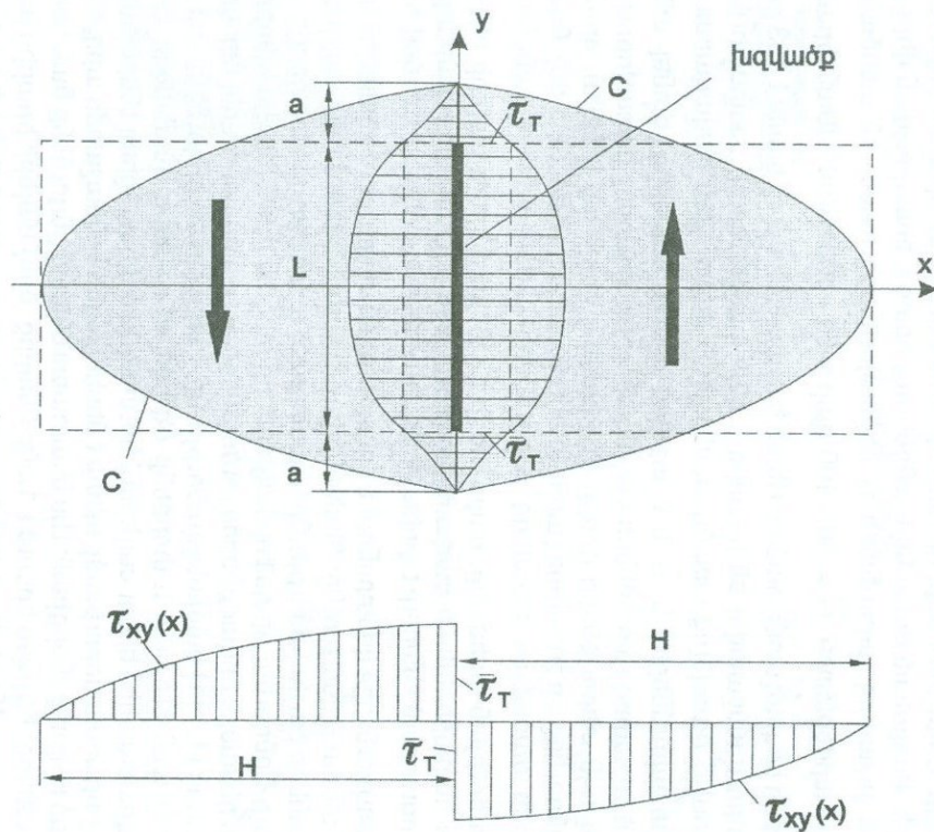
Նկ. 1.50 Միջավայրի դեֆորմացման սխեմատիկ պատկերը (a) և սահքի լարումների բաշխվածությունը:
