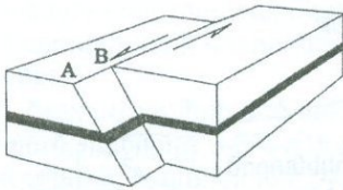
Չախակողմյան սահք
