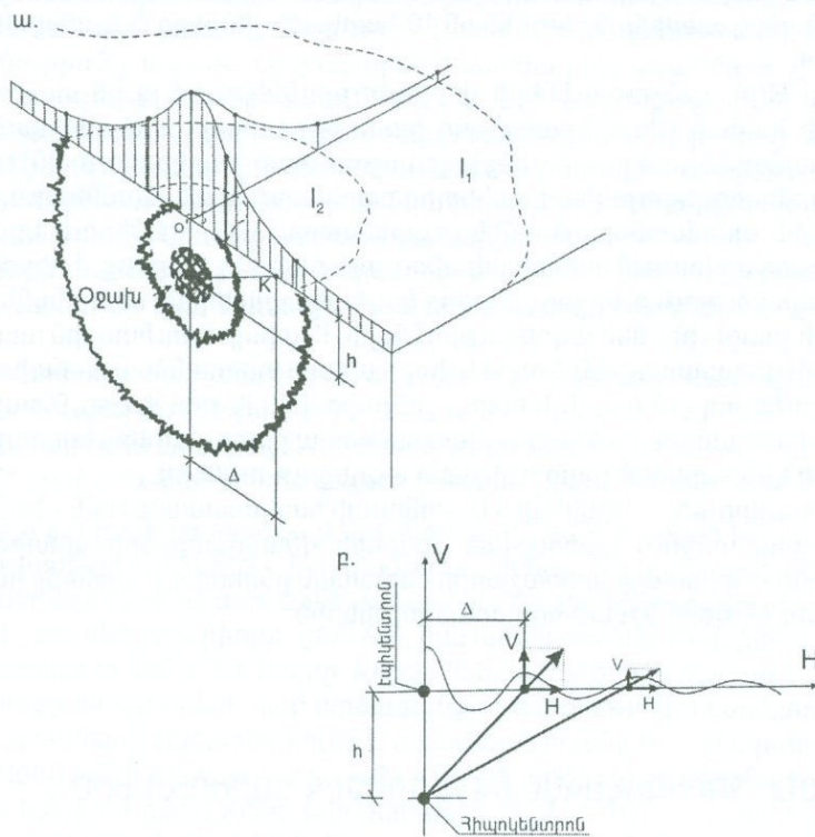
Նկ. 2.27 Երկրաշարժի օջախային գոտու (ա) և հորիզոնական ու ուղղաձիգ (բ) տատանումների կոմպոնենտների հարաբերության սխեմաները:
