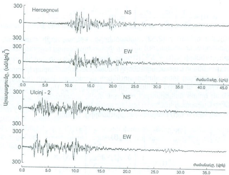
Նկ. 2.34 1979թ. ապրիլի 15-ի Սոնտեգրոյի երկրաշարժի հորիզոնական կոմպոնենտների արձանագրումները, գրանցված Hercegnovi և Ulcinj-2 կայաններում:
