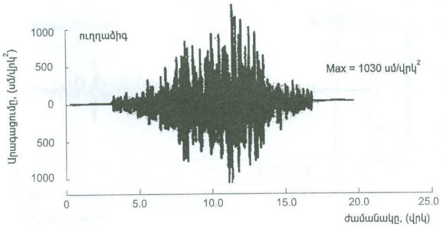
Նկ. 2.28.5 1976թ. մայիսի 17-ի Գազլիի երկրաշարժի արձանագրումը [129]:
