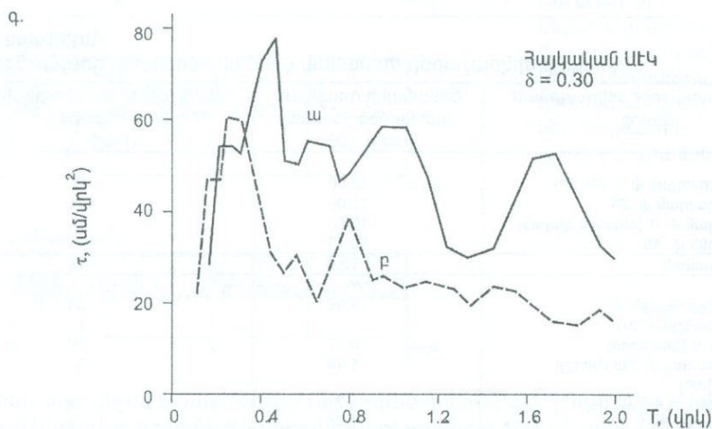
Նկ. 3.21 Սպիտակի երկրաշարժի ռեակցիայի սպեկտրները:
