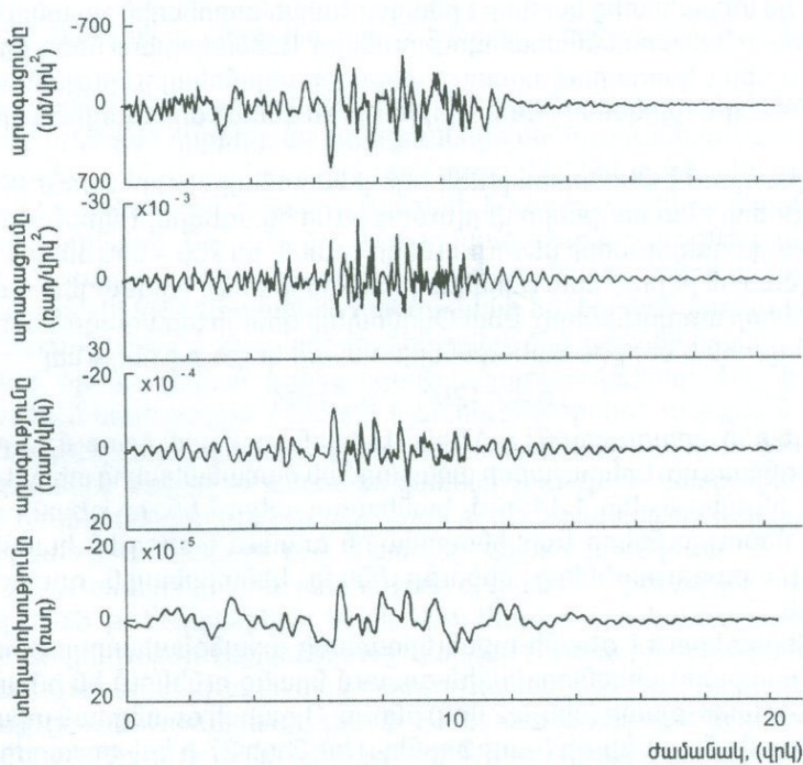
Նկ. 2.37 Գրունտի սինթետիկ քսելերոգրամը և նրանից ստացված գրունտի պտտական շարժման պարամետրերը [115]:
