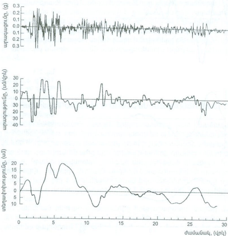
Նկ. 2.2 1940թ. մայիսի 18-ին Էլ-Ցենտրոյի երկրաշարժի քսելերոգրամը և նրանից ստացված վելիսոգրամը և սեյսմոգրամը [39]:
