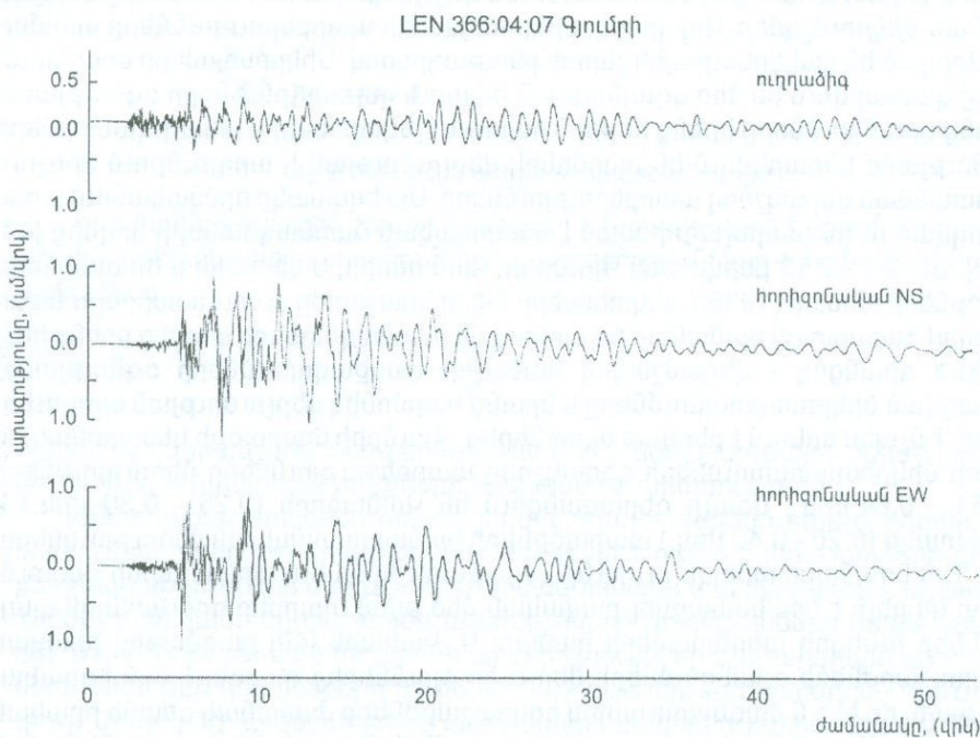
Նկ. 2.6 1988թ. դեկտեմբերի 31-ի աֆտերշոկի գրանցումները կարճր գրունտի վրա՝ Ջրաշենում (DZH) և փուխր գրունտի վրա՝ Լենինականում (LEN) [81]:
