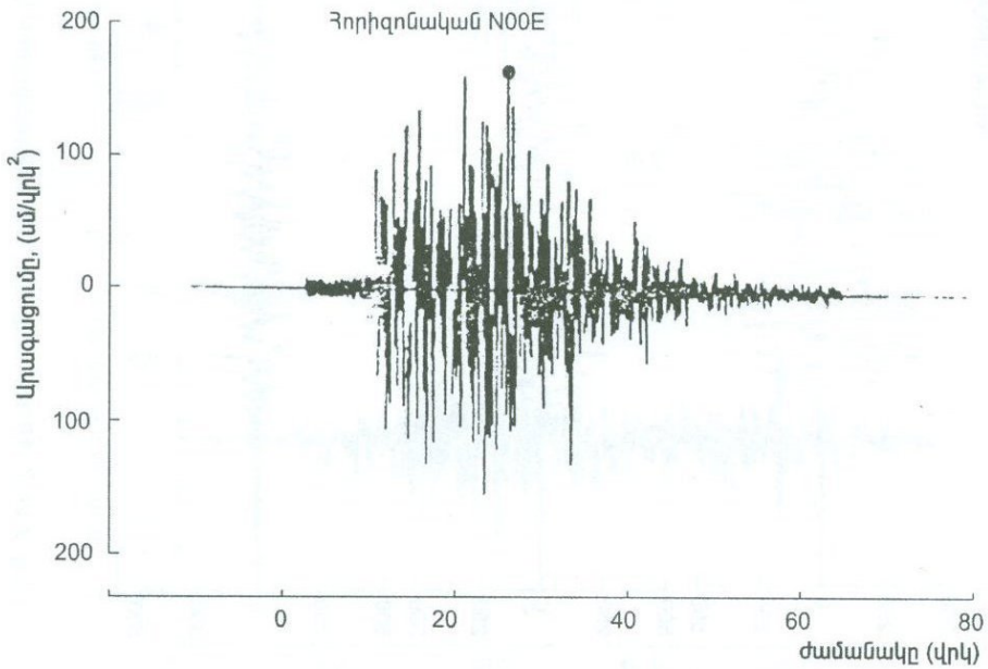
Նկ. 2.28.8 1985թ. սեպտեմբերի 19-ի Մեքսիկայի երկրաշարժերի աքսելերոգրամները [148]:
