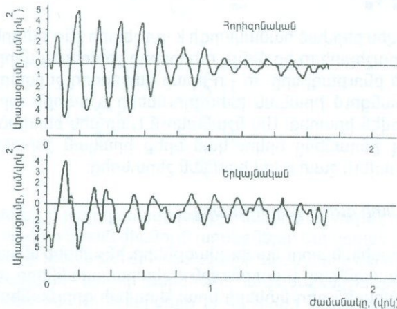
Նկ. 2.15 1973թ. Յունիսի 16-ի Երևանյան երկրաշարժի աքսելերոգրամը [59] (ԻՍԶԿ No. 1 բազալտներ, Երևան, Ահարոնյան 3. Հայսեսյան զհի):
