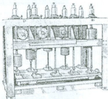
գ. АНС (ИГИС) տիպի սեյսմոմետր
