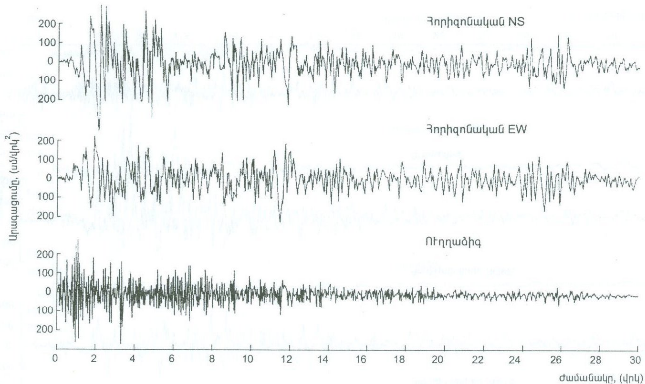
Նկ. 2.28.1 1940թ. մայիսի 18-ի ել-Ցենտրոյի երկրաշարժի եռակոմպոնենտ արժեքերի գրանցումները [137]:
