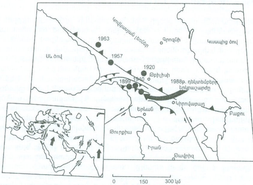
Նկ. 3.6 Սպիտակի երկրաշարժի տեկտոնական դրությունը [92]:
