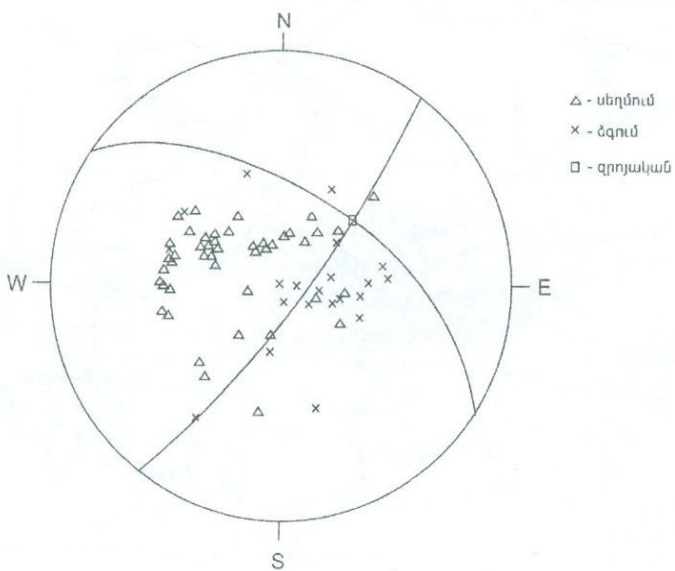
Նկ. 3.10 Սպիտակի երկրաշարժի օջախի ֆոկալ մեխանիզմը [92, 136]:
