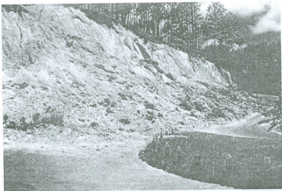
Նկ. 1.5 Երկրաշարժի հետևանքով առաջացած սողանք [143]:
