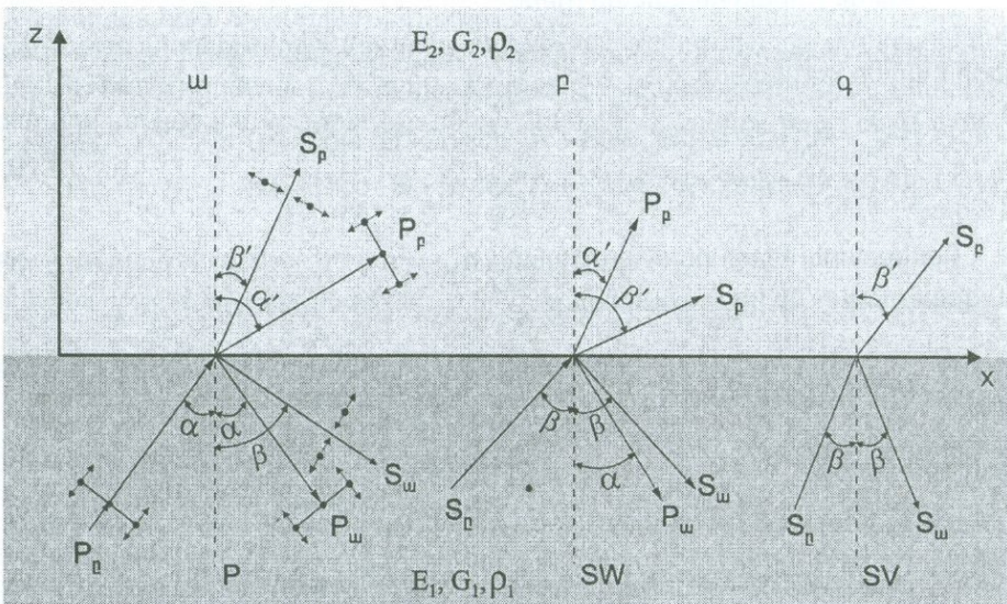
Նկ. 1.39 Սեյսմիկ ալիքների բեկումը և անդրադարձումը:
