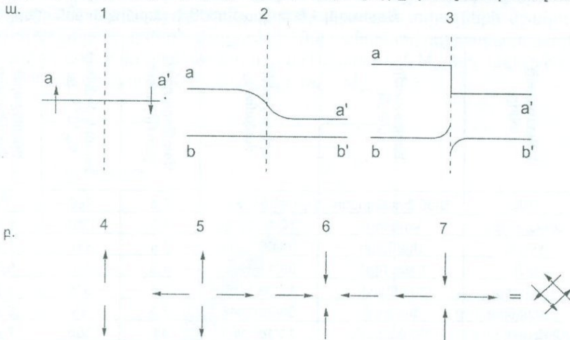
Նկ. 1.47 Առաձգական տաքցի Ռեյլիի մոդելը (ա) և երկրաշարժի առաջացման կետային աղբյուրների (4-7) տարբեր տիպերը (բ) [49] 1-դեֆորմացիաները բացակայում են 2-կուտակված դեֆորմացիաների դեպքում 3-խզվածքով տեղաշարժ առաջացումից հետո:
