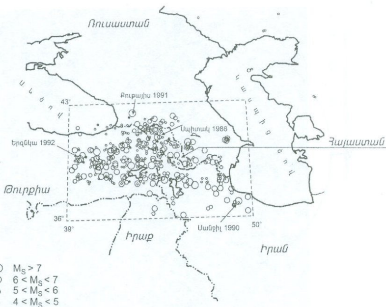
Նկ. 3.8 Մ.թ. 139 մինչև 1992 թվականը Հայկական լեռնաշխարհում ու հարակից շրջաններում տեղի ունեցած պատմական երկրաշարժերը [152]:
