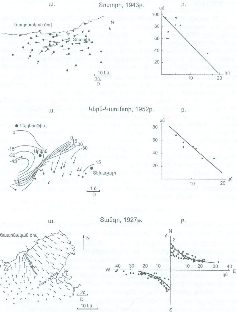
Նկ. 1.49 Երկրաշարժերի ժամանակ III դասի տրիանգուլյացիայի արդյունքում տեղամասերի հորիզոնական տեղաշարժերը (ա) և խզվածքին զուգահեռ ուղղությամբ տեղաշարժերի նվազումը (մ.) համապատասխանաբար Տոտորի, Կերն-Կաունտիի և Տանգոյի երկրաշարժերի դեպքում [43]:
