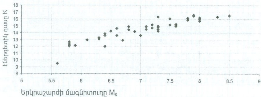
Նկ. 1.52 Երկրաչափների էներգետիկ դասի կախվածությունները երկրի մակերևույթի վրա խզվածքի երկարությունից, հարաբերական տեղաշարժի միջին մեծությունից, խզվածքի խորությունից և մագնիտուդի մեծությունից:
