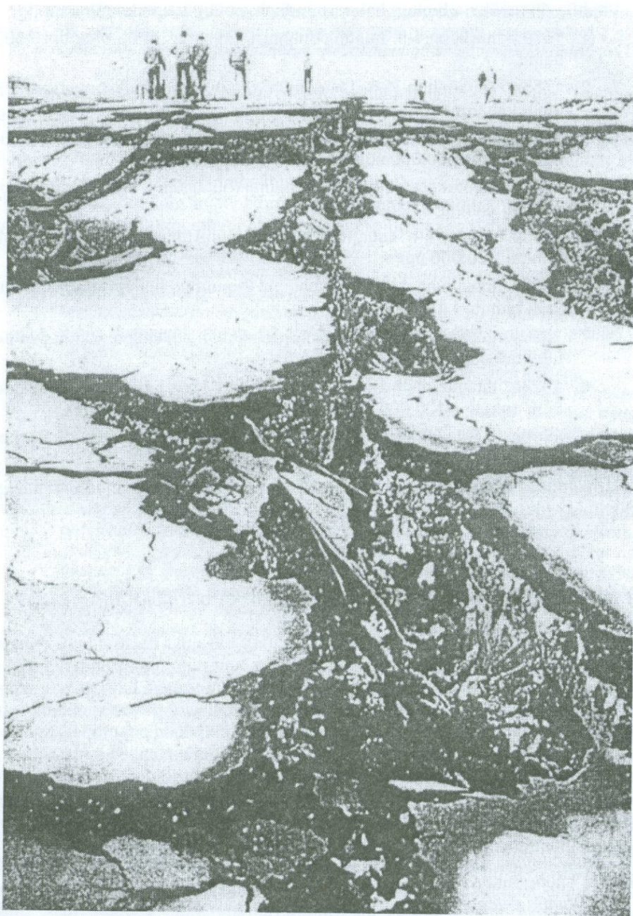
Նկ. 1.1 ճաքեր (պատռվածքներ) ճապոնական Նիիգատա քաղաքի շրջակայքում 1964թ. հունիսի 16-ի երկրաշարժից հետո [69]:
