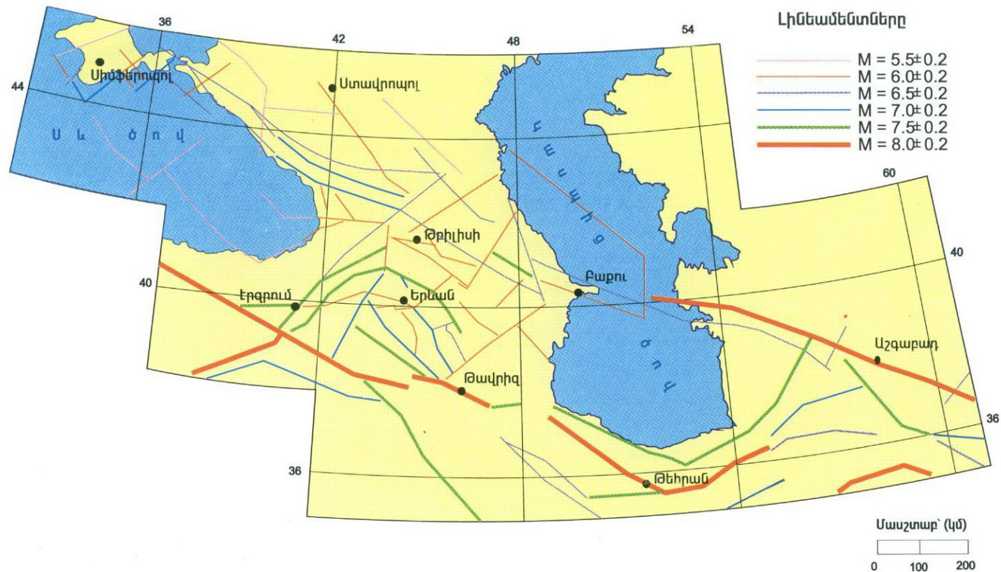
Նկ. 3.2 Կովկասյան տարածքի երկրաշարժերի օջախային գոտիների լիցենամենտային մոդել [74]
