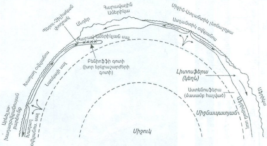
Նկ. 1.11 Երկրագնդի կառուցվածքը [23]:
