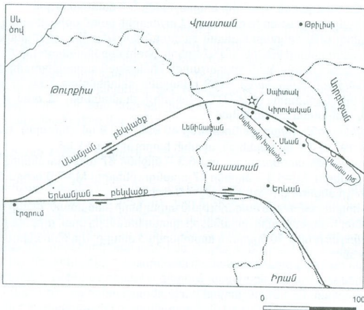
Նկ. 3.7 Ռեգիոնալ տեկտոնական քարտեզի վրա Սպիտակի երկրաշարժի տեղակայումը [136]:
