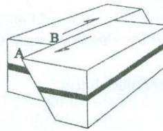
Աջակողմյան սահք
