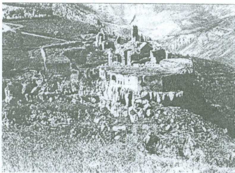
Նկ. 3.4 Տաթևի վանքահամալիրը 1931թ. Ջանգեզուրի երկրաշարժից առաջ և հետո:
