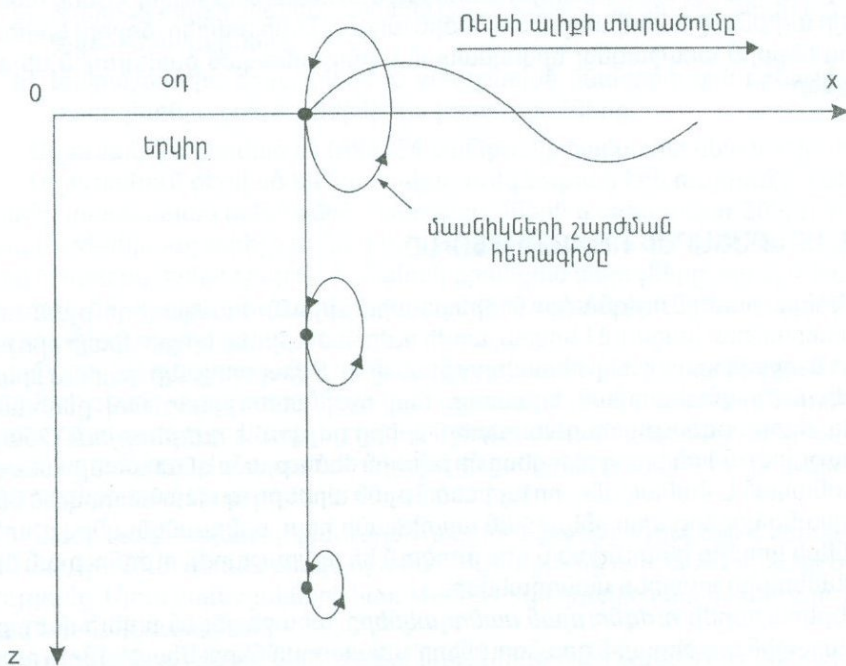
Նկ. 1.41 Ռելեի ալիքների տարածությունը [47]:
