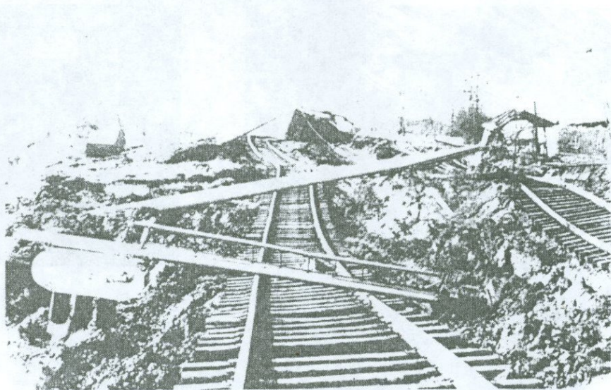
Նկ. 1.8 Երկաթգծերի ծոռվածքներ Սպիտակի երկրաշարժից՝ Նալբանդի շրջակայքում գետնի շրջիկացման պատճառով [151]:
