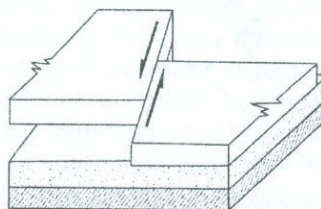
Չափոխված խզվածք
