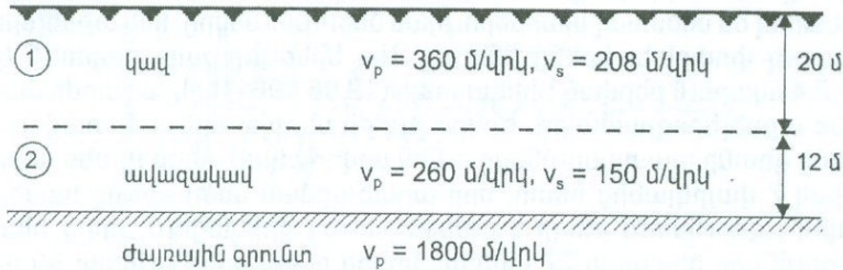
Նկ. 2.17 ԷԼ-Ցենտրոն կայանի գրանցման տեղամասի երկրաբանական կտրվածքը ըստ [40]:
