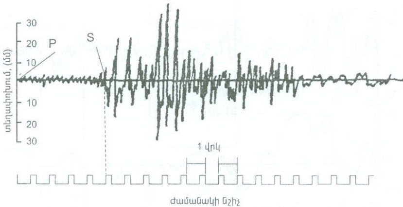
Նկ. 1.25 Միջին ուժգնության երկրաշարժի սեյսմոգրամը:
