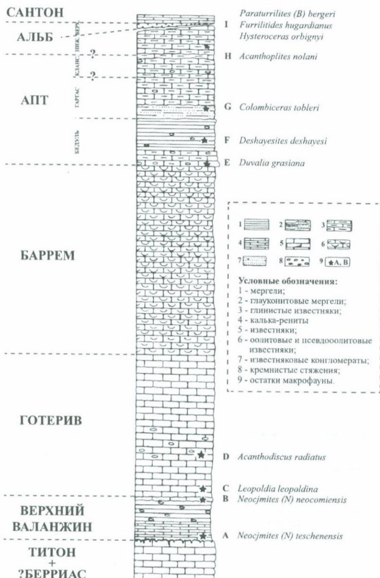
Рис. 4 – Разрез нижнего мела у Оросеи (восточное побережье Сардинии); по И. Видманну и И. Дени (Wiedmann, Deni, 1968, стр. II, фиг. 2)
