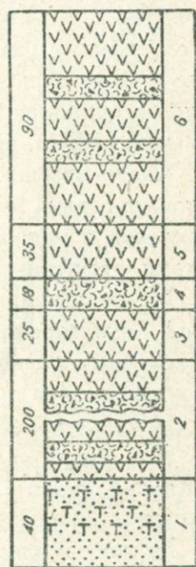
Рис. 5. Разрез верхнего байоса окрестно- стей г. Кафан.
