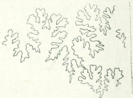
Рис. 66. Лопастная линия Barremites difficilis d'Orb. при В=21 мм (обр. 1020/7).
