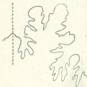
Рис. 59. Лопастная линия Salfeldiella milaschewitschi Kar. при В=14 мм (обр. 1020/15).
