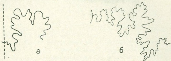
Рис. 70. Лопастная линия Barremites charrierianus d'Orb. а) при B=6 мм, б) при B=7,5 мм (обр. 1020/12).
