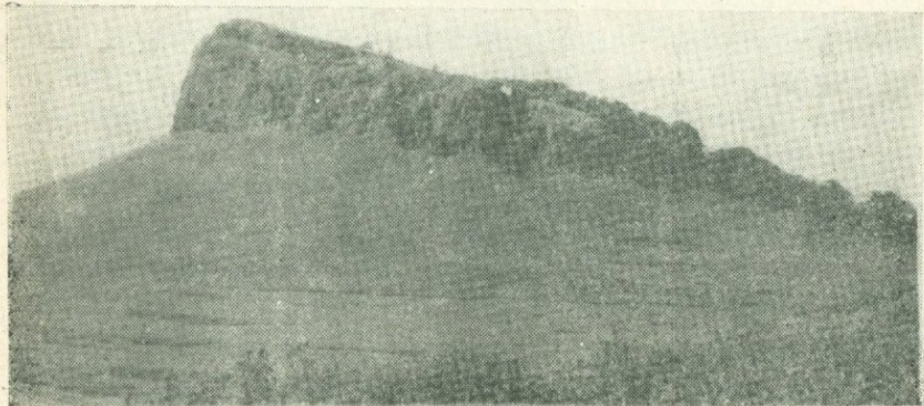
Рис. 42. Известняки неокома на вершине г. Кяпаз.
