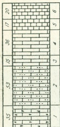
Рис. 37. Разрез баррема на г. Кармир-ванк.
