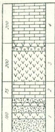
Рис. 18. Разрез тапасар-кар- мракарской свиты на г. Кыки.
