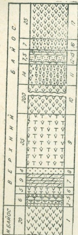
Рис. 6. Разрез верхнего байоса у с. Арфик.
