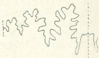
Рис. 72. Лопастная линия Holcodiscus geronimae Негт. при T=3,2 мм (обр. 1020/1).
