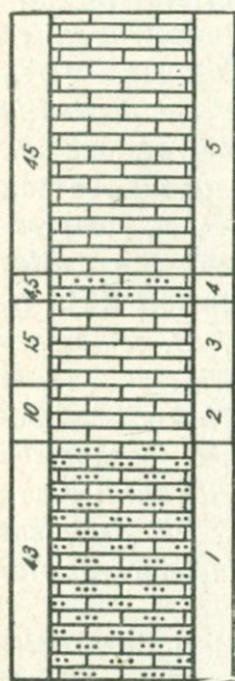
Рис. 35. Разрез баррема у с. Арцваник.
