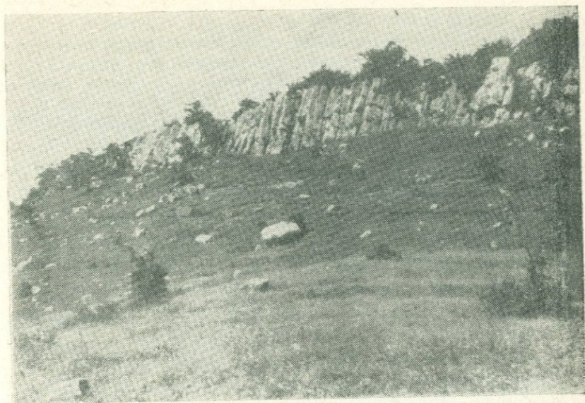
Рис. 33. Известняки агаракской подсвиты у перевала Кармракар.
