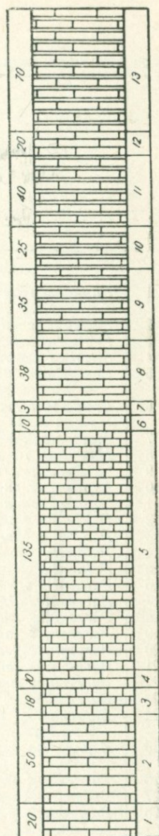
Рис. 47. Разрез карбонатной свиты неокома на г. Хуступ.
