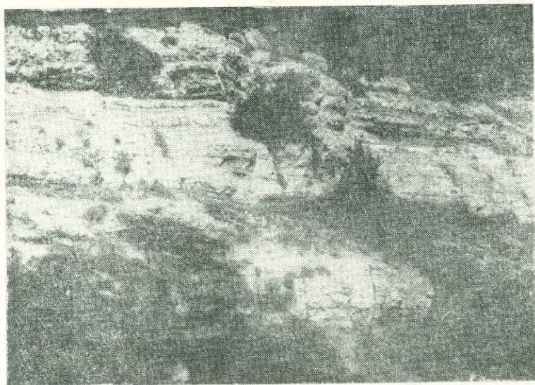
Рис. 20. Песчаники и известняки пачек 19 и 20 западнее перевала Кармракар.
