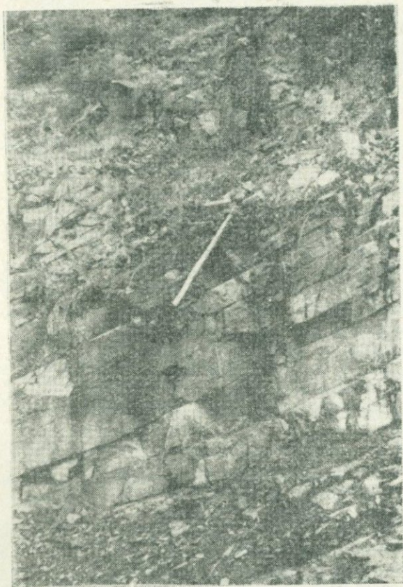
Рис. 23. Тонкая трещиноватость в фиолетовых порфиритах хуступ-чиманской толщи у с. Шикахох.
