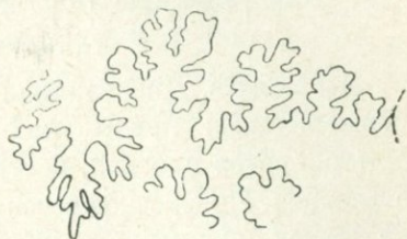
Рис. 71. Лопастная линия Barremites compsense Kil. при B=11,5 мм (обр. 1020/13).
