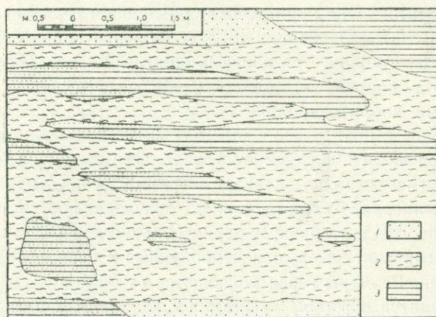
Рис. 58. Взаимоотношение туфопесчаников и сланцев у восточной окраины с. Сваранц (план): 1—наносы; 2—сланцы; 3—туфопесчаники верхнего конька.
