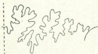
Рис. 68. Лопастная линия Barremites tenuicinctus Sar. et Schönd. при В=5 мм (обр. 1020/10).
