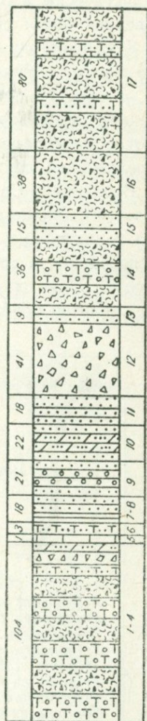
Рис. 57. Разрез верхнего коньяка ущелья р. Агандзугет.
