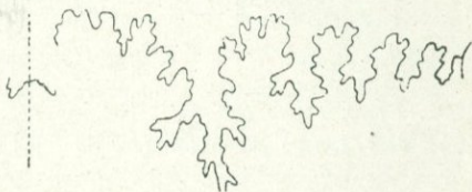
Рис. 67. Лопастная линия Barremites falloti Kil. при B=8 мм (обр. 1020/8).
