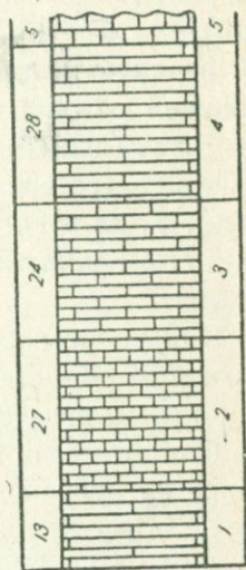
Рис. 45. Разрез карбонатной свиты неокома на г. Карентак.
