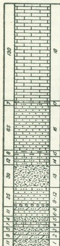
Рис. 53. Разрез верхнего турона (?)-нижнего коньяка восточнее с. Сваранц.
