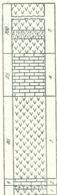
Рис. 21. Разрез титона—среднего валанжина района сс. Нор-Арачадзор.
