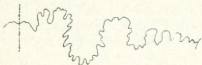
Рис. 62. Лопастная линия Pulchellia sauvageani Her m. при V=8 мм (обр. 1020/3).
