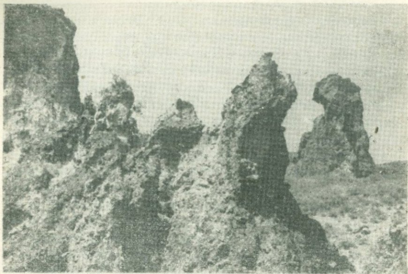
Рис. 2 Выходы пород горисской вулканогенно-обломочной свиты („каменные грибы“) между сс. Шинугайр и Хот.
