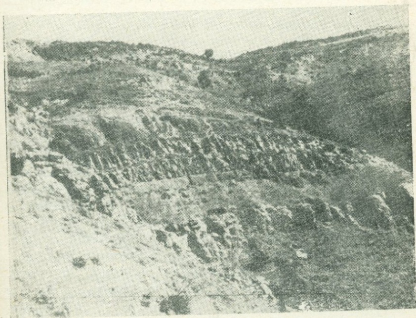
Рис. 28. Печки известняков в гейяльской вулканогенной свите у с. Гейял.
