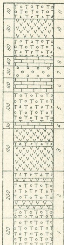
Рис. 9. Разрез лузитана — кимериджа у с. В. Вачаган.
