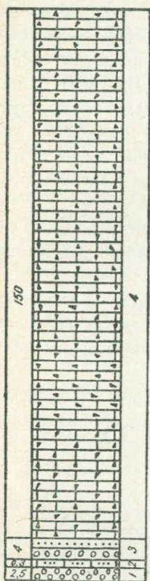
Рис. 29 Разрез верхнего валанжина—готерива у с. Агарак.
