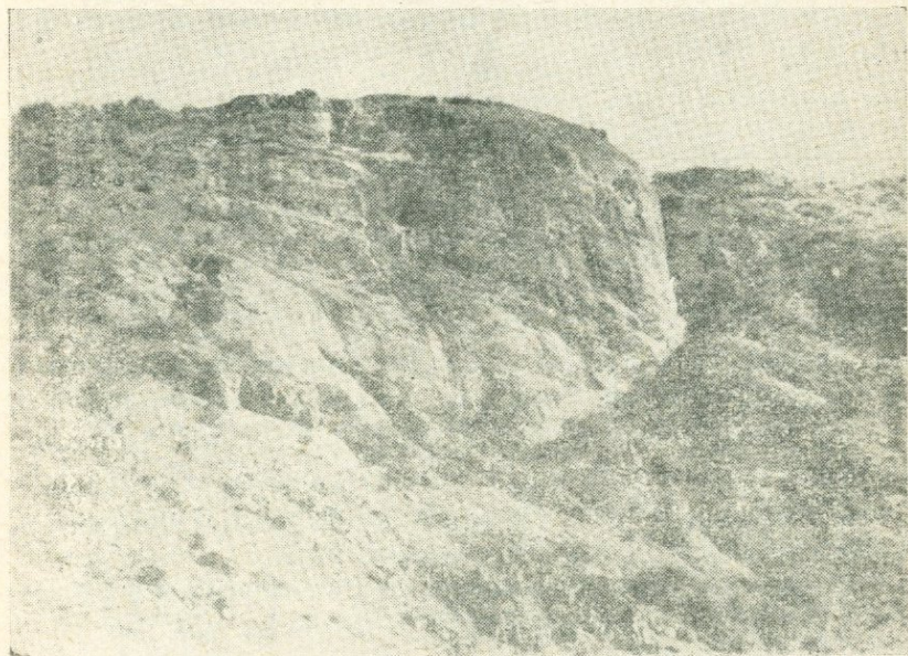
Рис. 8. Скала «Урац-кар» (восточнее с. Гехануш). Туфоконгломераты лузитана—кимериджа.
