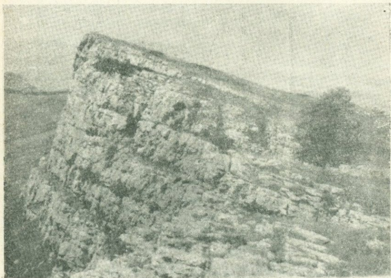
Рис. 43. Верхняя часть известняков вершины г. Кяпаз.
