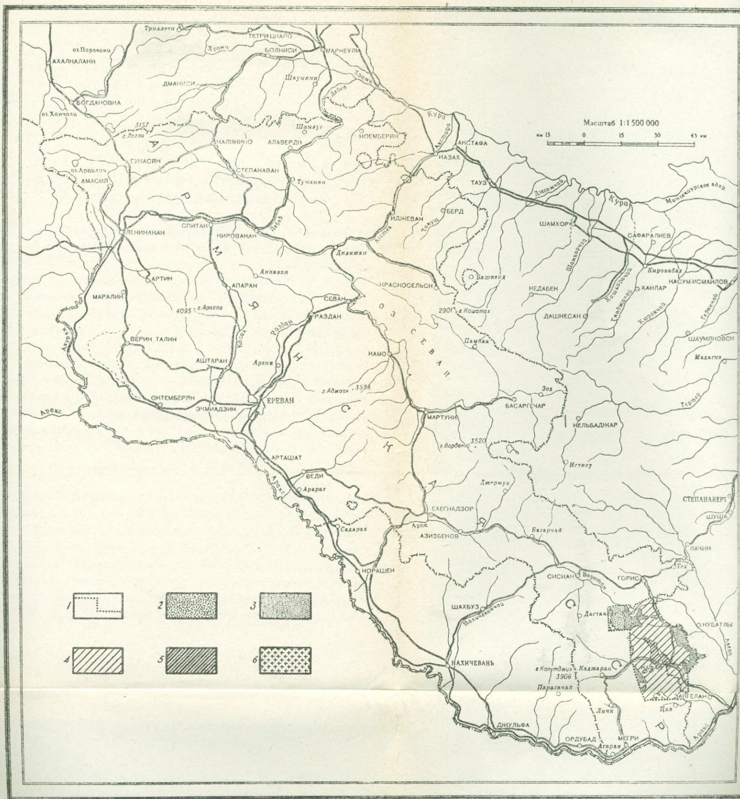
Рис. 1. Схема распространения юрских меловых отложений в юго-восточном Зангезуре.
