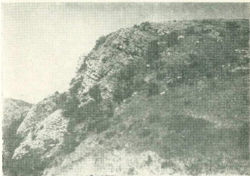
Рис. 36. Известняки баррема на г. Кер-кар (у с. Ариваник).
