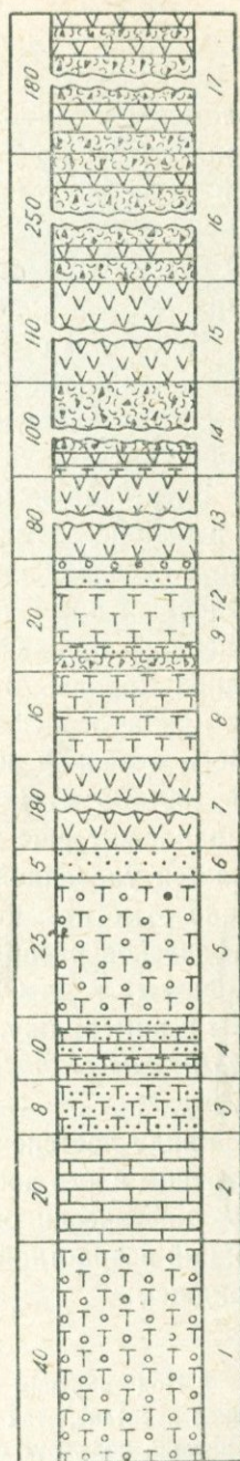
Рис. 12. Разрез лузитана—кимериджа у с. Антарашат.
