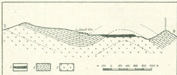
Рис. 40. Взаимоотношение свит известняков и вулканогенных пород в районе с. Давид-бек. 1— четвертичные андезитобазальты; 2— зейвинская свита известняков (верхний валанжин—баррем); 3— тапасар-кармакарская вулканогенная свита (титон—средний валанжин).
