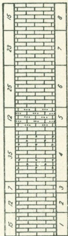
Рис. 39. Разрез известняков неокома у с. Да- вид-бек.
