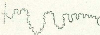
Рис. 65. Лопастная линия Pulchellia armenica Насов, при B=11 мм (обр. 1020/6).
