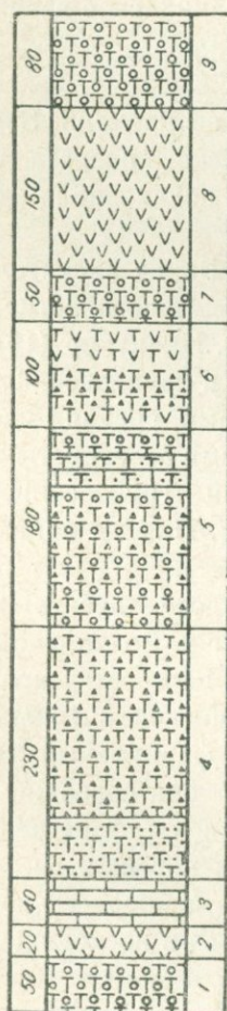
Рис. 10. Разрез лунитана — кимериджа района сс. Ачхлу—Шгар- джик.
