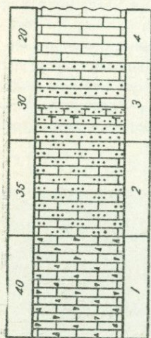
Рис. 56. Разрез верхнего турона (?) - нижнего коньяка в районе с. Татев (выс. 1756,8).
