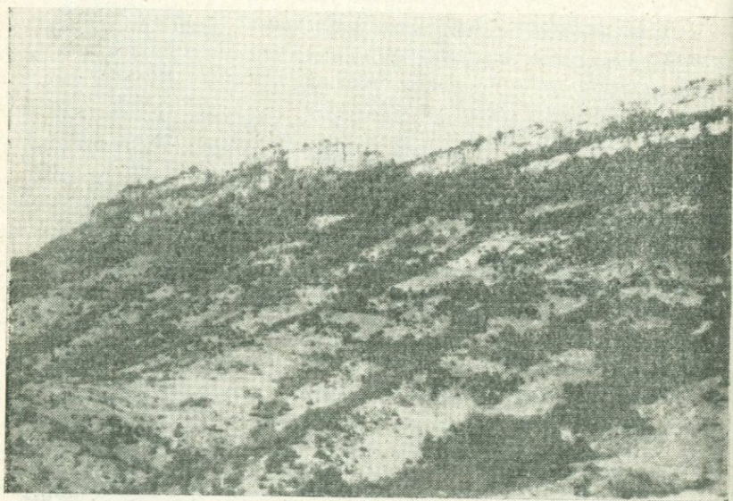
Рис. 31. Свита известняко в неокома (верхний карниз) у с. Арцваник.
