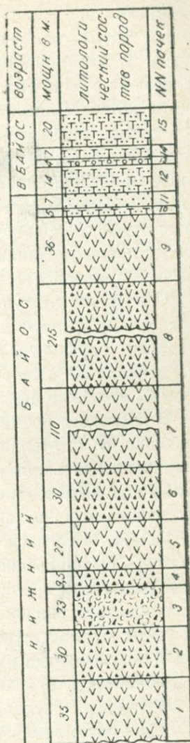
Рис 4. Разрез нижнего байоса ущелья р. Куртамяк.
