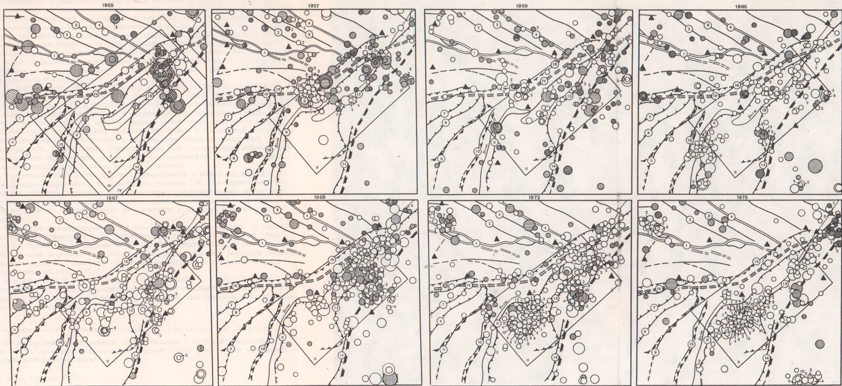
Рис. 5. Карты эпицентров землетрясений за 1955-1973 гг. I-IV - контуры вокруг водохранилища; V - контур водохранилища Усл. обозн. см. на рис. 1. Цифры со стрелкой указывают количество землетрясений
