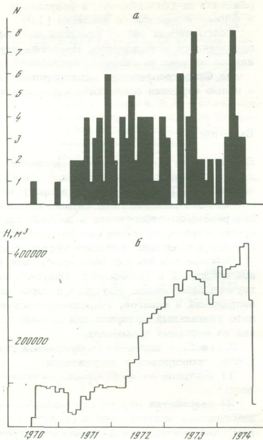
Рис. 7. Корреляция количества землетрясений N (а) с объемом жидкости H , закаченной в пласт (б)
