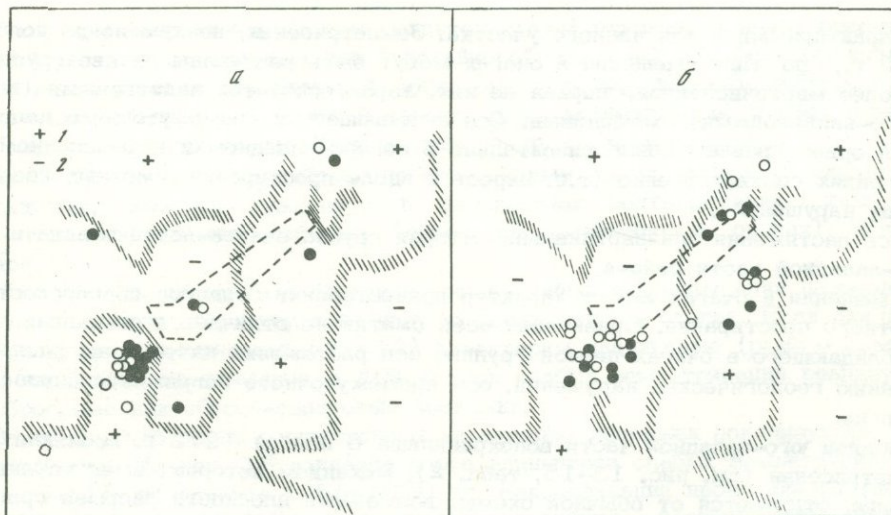
Рис. 17. Карты эпицентров землетрясений, возникших в 1971 (а) и в 1972 гг. (б)
