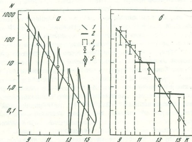
Рис. 1. Схема к расчетам графиков повторяемости
