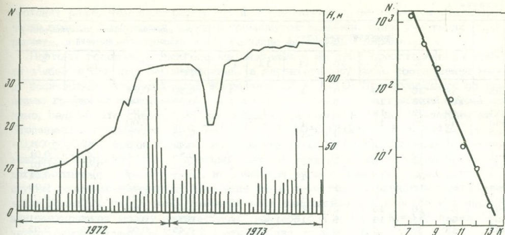
Рис. 8. Декадные суммы землетрясений N ( K \geq 7 ) за 1972–1973 гг. и изменение во времени уровня воды H в водохранилище
