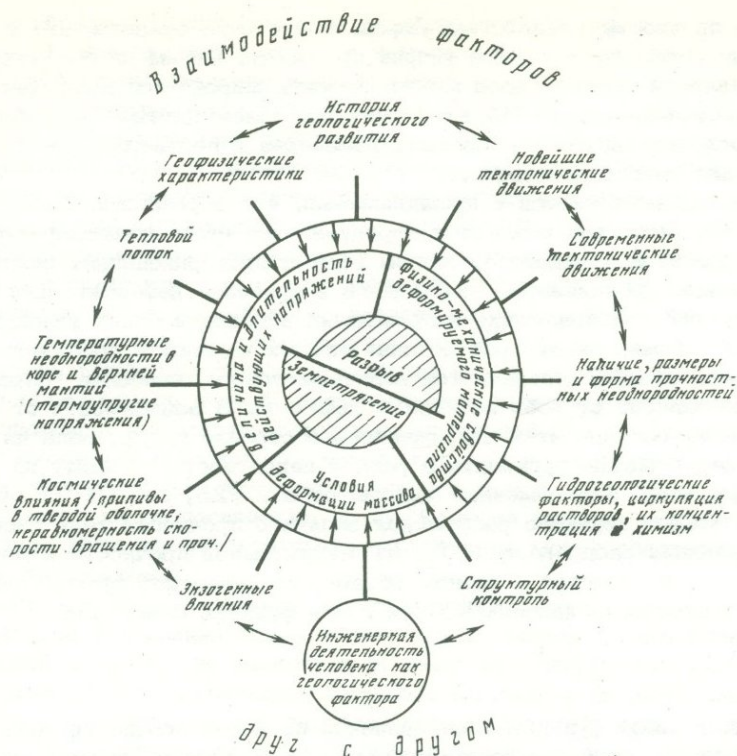
Рис. 3. Стохастическая модель сейсмотектонических связей
