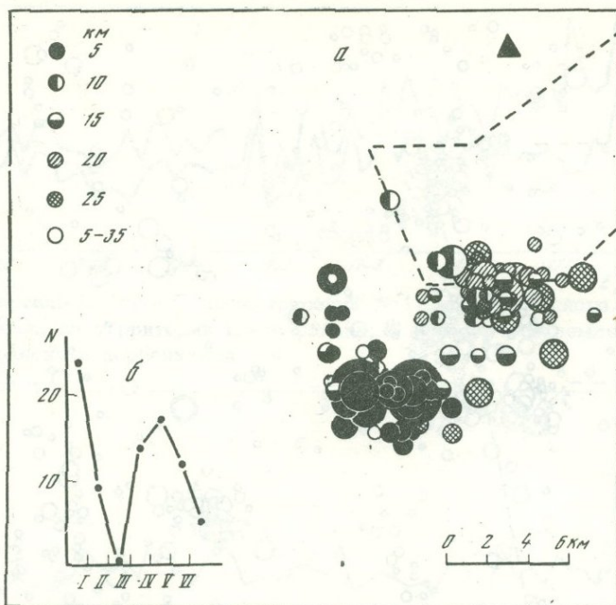
Рис. 13. Карта эпицентров землетрясений (а), возникших в течение 35 дней (I-VII - пятидневки) после толчка с K = 12 , и график суммы землетрясений N на каждую пятидневку (б)
