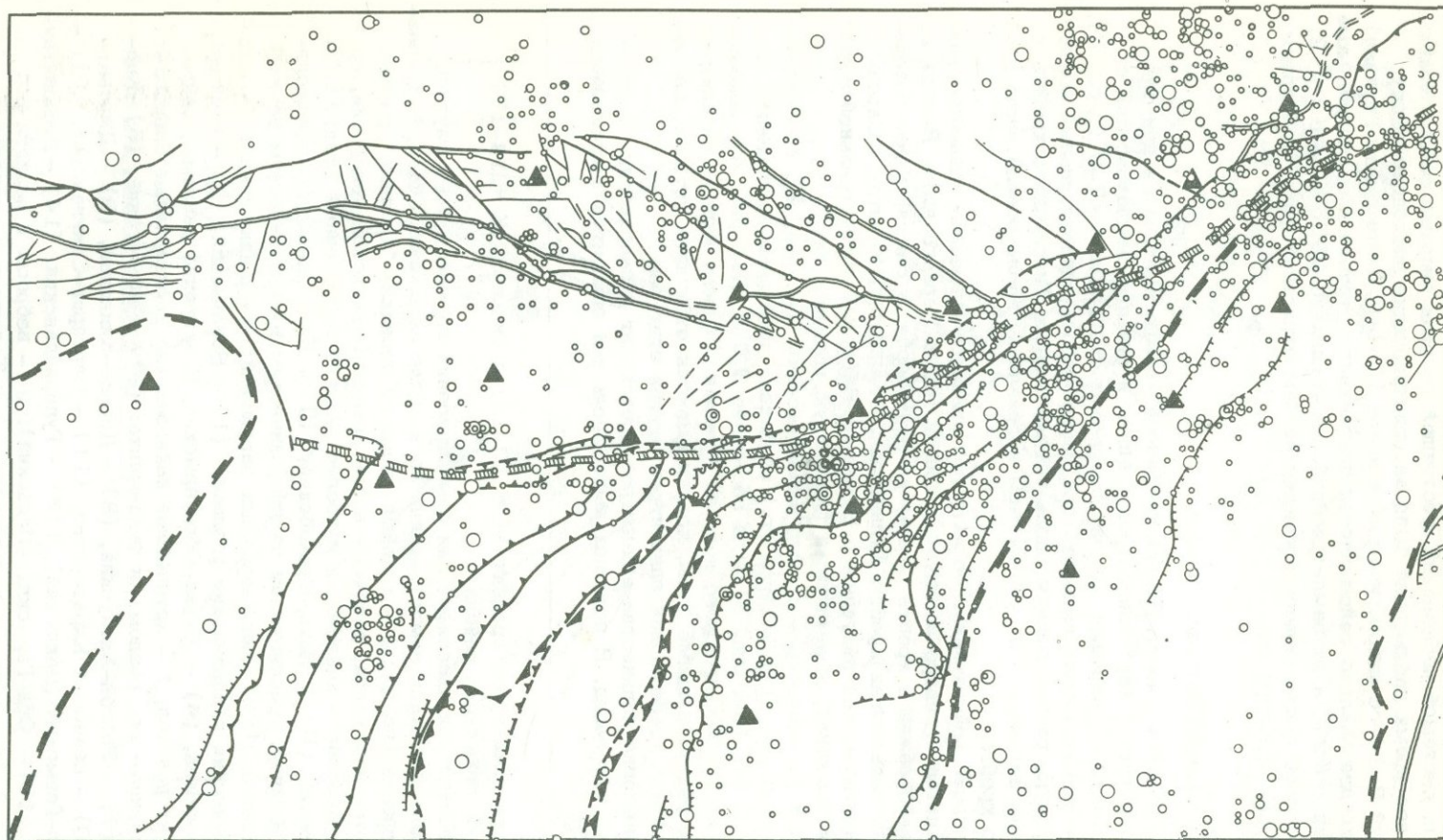
Рис. 2. Карта эпицентра слабых ( K = 7-9 ) землетрясений Вахшского района за 1955-1962 гг. Усл. обоз. см. на рис. 1
