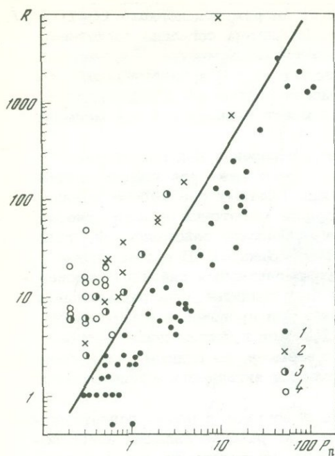
Рис. 2. Отношения амплитуд релеевских R и продольных волн P_n для подземных ядерных взрывов различной мощности
