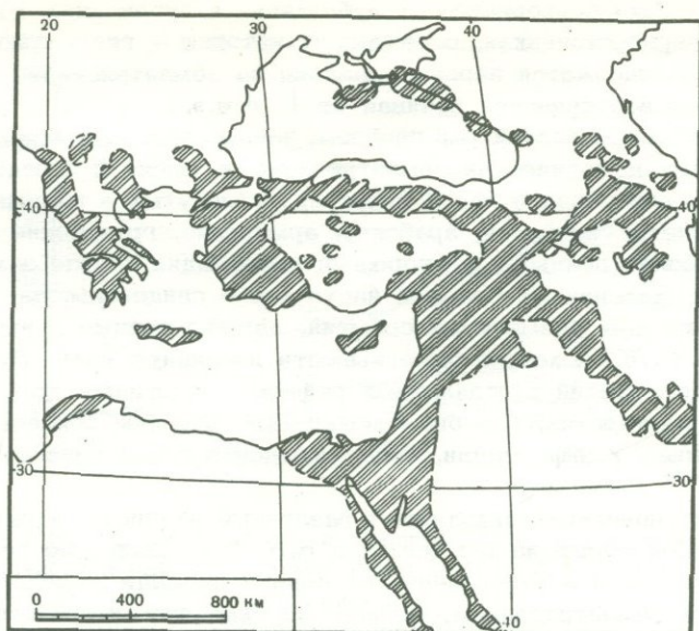
Рис. 1. Карта распределения исторических землетрясений
