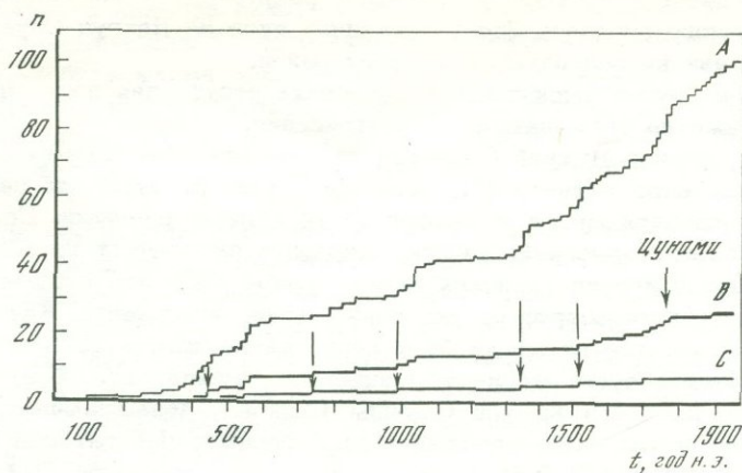
Рис. 2. Сейсмическая активность за историческое время для района Стамбула (по Н.Н. Амбразею)
