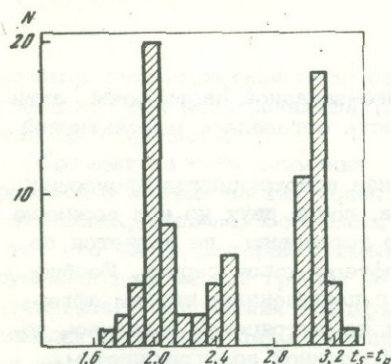
Рис. 14. Гистограмма разности времени прихода поперечной и продольной волн ( t_s - t_p ) на сейсмическую станцию Лянгар
