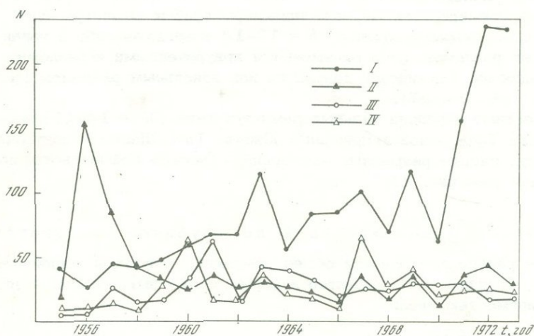
Рис. 6. Годовые суммы землетрясений N ( K \geq 7 ), возникающих вокруг водохранилища на площадках разной величины
