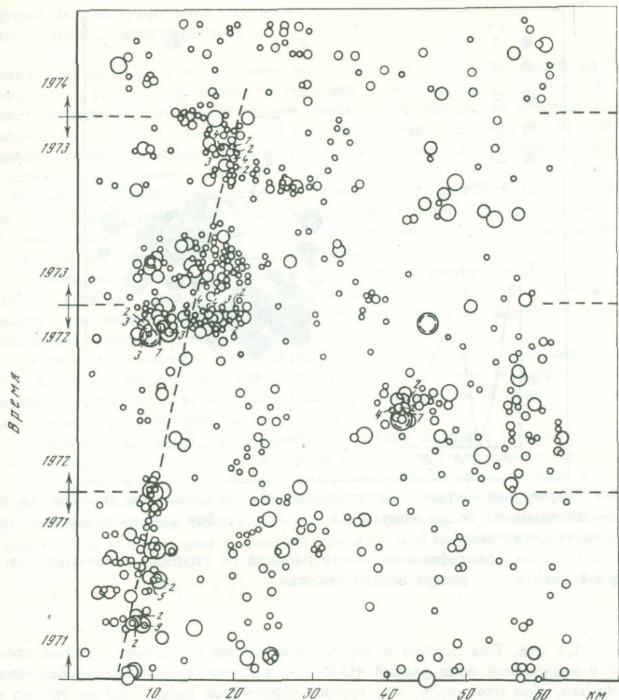
Рис. 12. Пространственно-временное распределение землетрясений вблизи водохранилища
