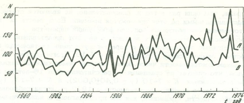
Рис. 10. Квартальные суммы землетрясений N ( K \geq 7 ) Вахшского района А – возникших на территории всего района; Б – без учета землетрясений, возникших в районе водохранилища
