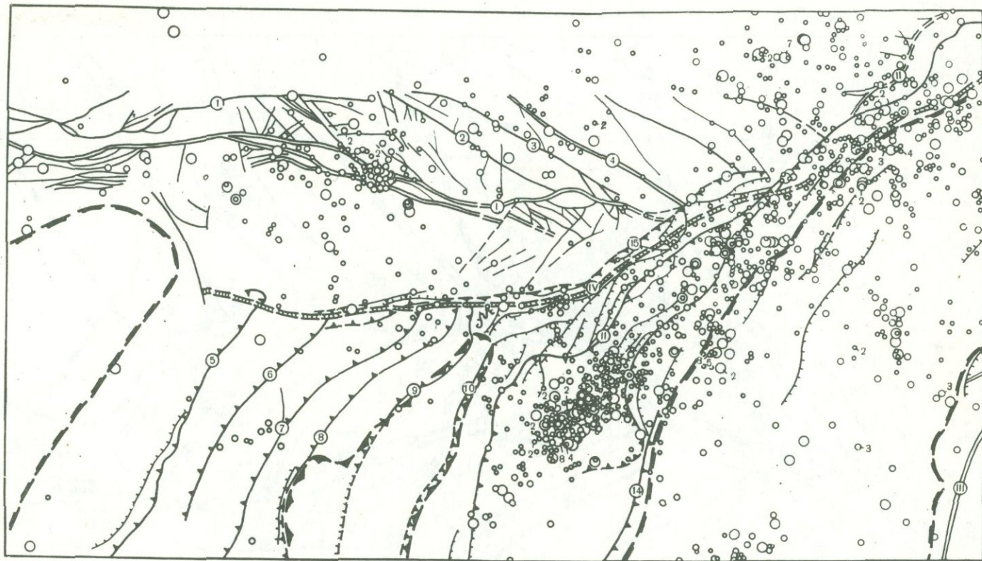
Рис. 4. Карта эпицентров слабых ( K = 7-9 ) землетрясений Вахшского района за 1971 г. - июнь 1974 г. Усл. обозн. см. на рис. 1
