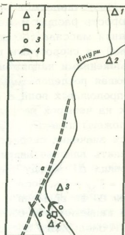
Рис. 1. Схема расположения пунктов геофизических наблюдений в р-не строительства Ингури ГЭС
