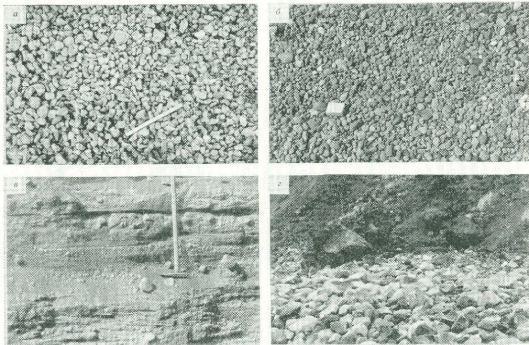
РИС. 35. Тейфроида:
