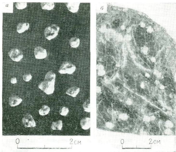
РИС. 4. Сферолиты: а — извлеченные сферолиты; б — сферолиты в перлите
