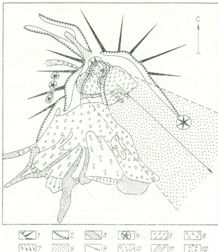
РИС. 65. Отложения вулкана Шивелуч извержения 12 ноября 1964 г. (по Г. С. Горшкову, Ю. М. Дубику [36]):
