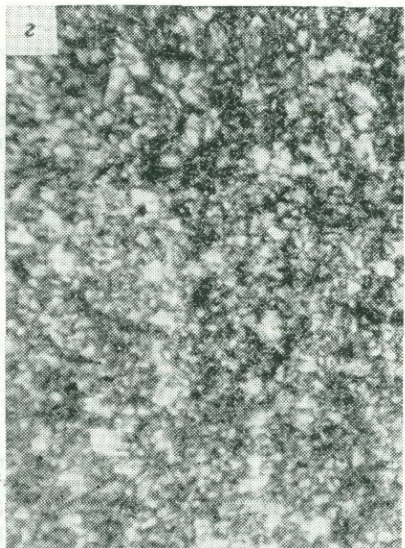
РИС. 20. Структуры
