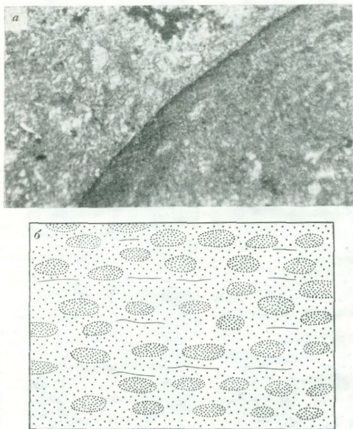
РИС. 17. Пизолитовая текстура под микроскопом (а) и зарисовка образца (б), девон Южного Казахстана
