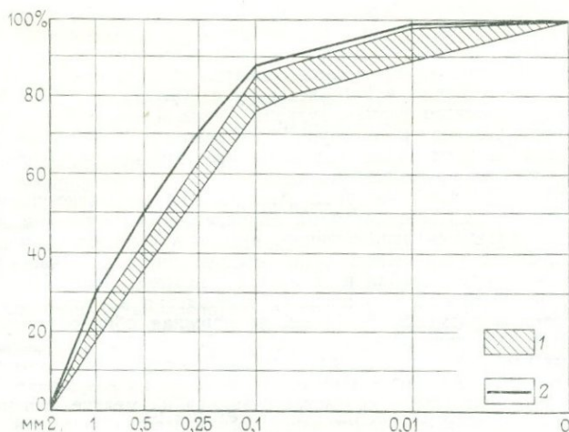
РИС. 67. Крупность материала наполнителя агломеративного пирокластического потока вулкана Безымянного извержения 1956 г.:
