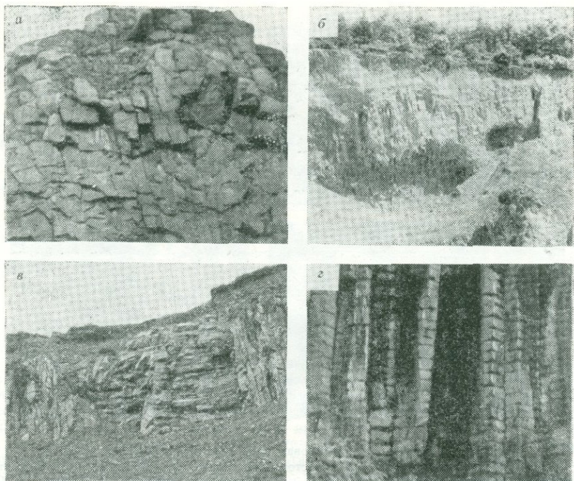
РИС. 13. Виды отдельности:
