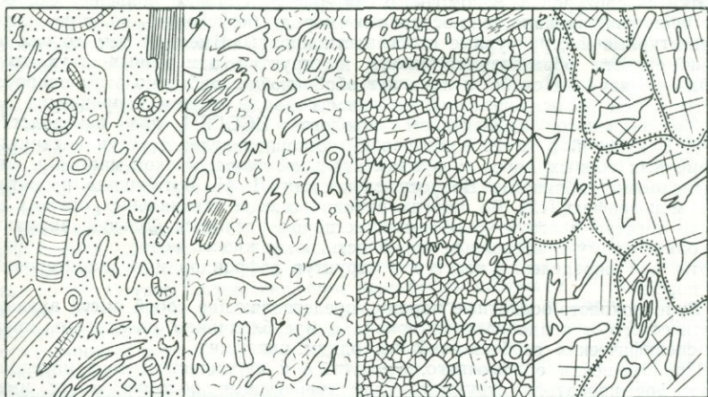
РИС. 23. Структуры смешанных пород: а — алевритовая, туфодиатомитовая структура, Приморье; б — туфотерригенная структура в псаммитовом витрокластическом туфопесчанике, о. Парамушир, Курильские острова; в — псаммитовая туфокarbonатная структура в туфоизвестняке, Закавказье; г — псаммитовая туфоглауцидная структура, Карпаты
