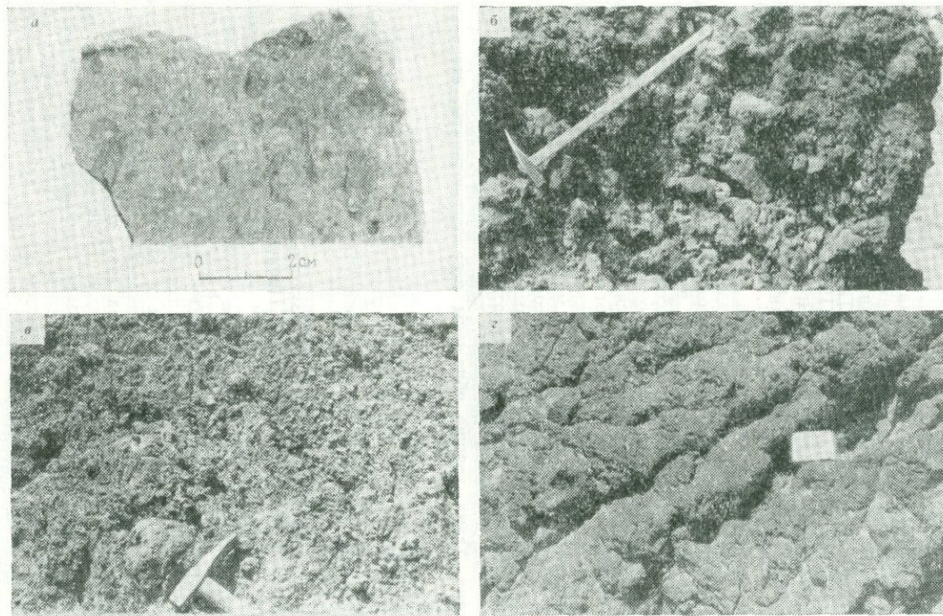
РИС. 32. Спекшиеся туфы:
