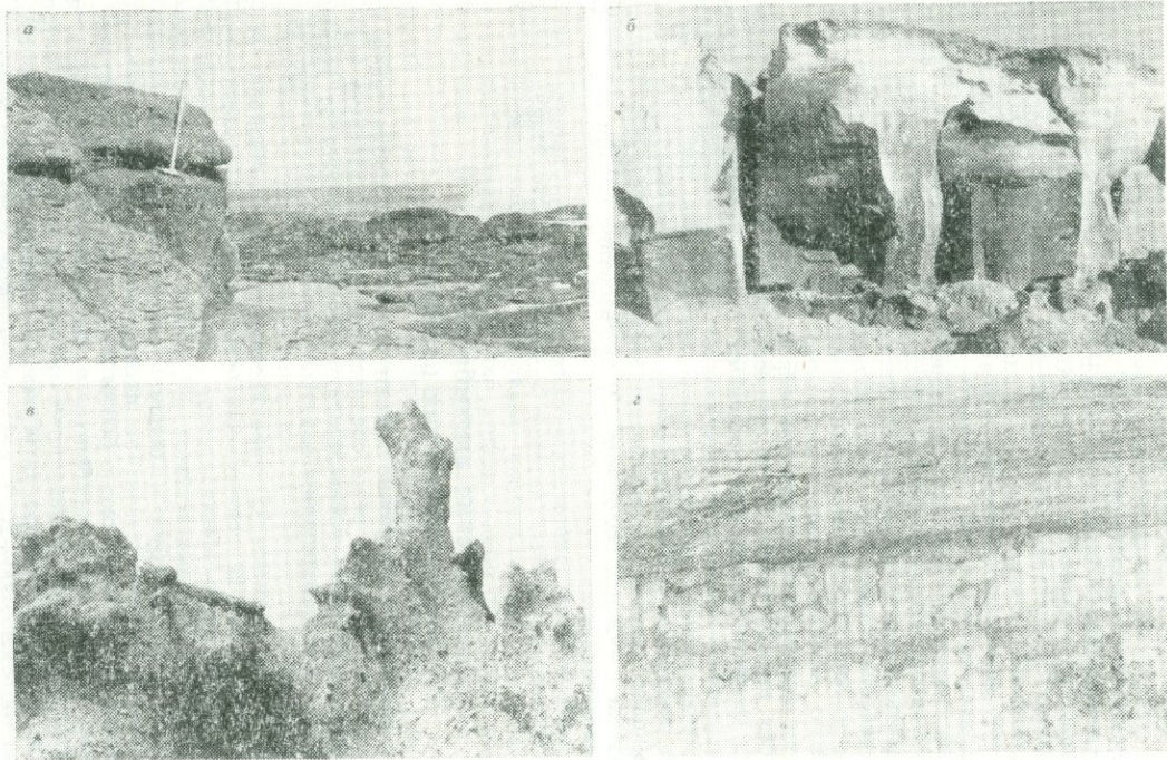
РИС. 63. Отложения пирокластических потоков:
