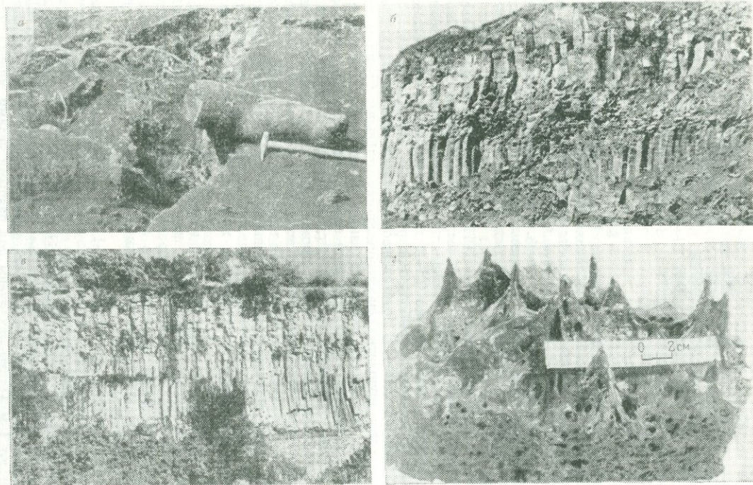
РИС. 42. Отдельность и текстурные особенности лав:
