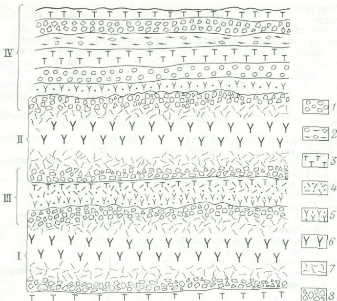
РИС. 73. Модель лавово-вулканокластических образований. I—II нижний и верхний лавовые потоки; III — горизонт лавокластического материала; IV — перекрывающие вулканогенные образования, обычные для промежуточной зоны:
