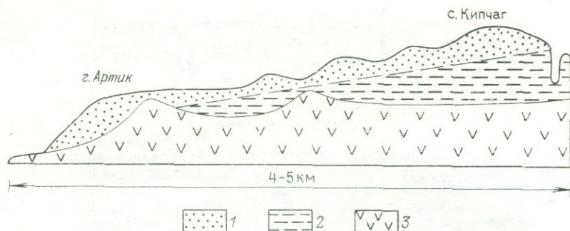
РИС. 47. Строение дацитового потока в районе г. Артик [105]: 1 — арктическая туфолова; 2 — щелочной дацит; 3 — догуфовое основание
