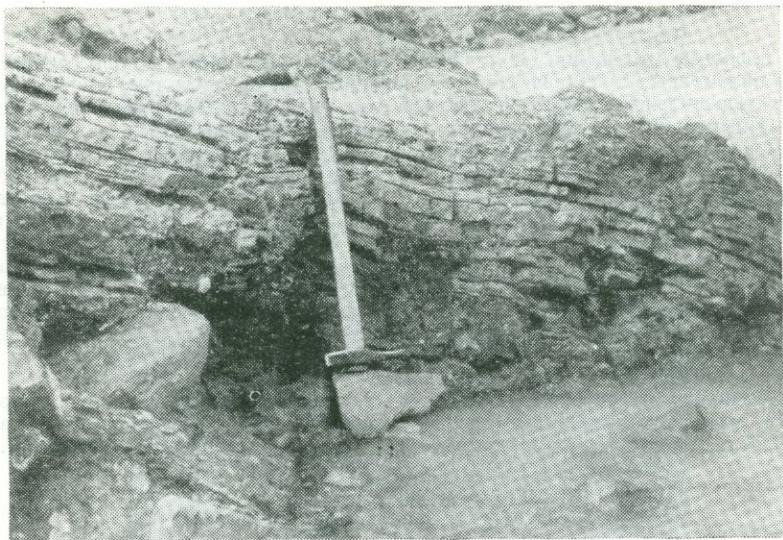
Рис. 59. Образование тонкослоистых отложений серы в кратерном озере вулкана Эбеко на о. Парамушир
