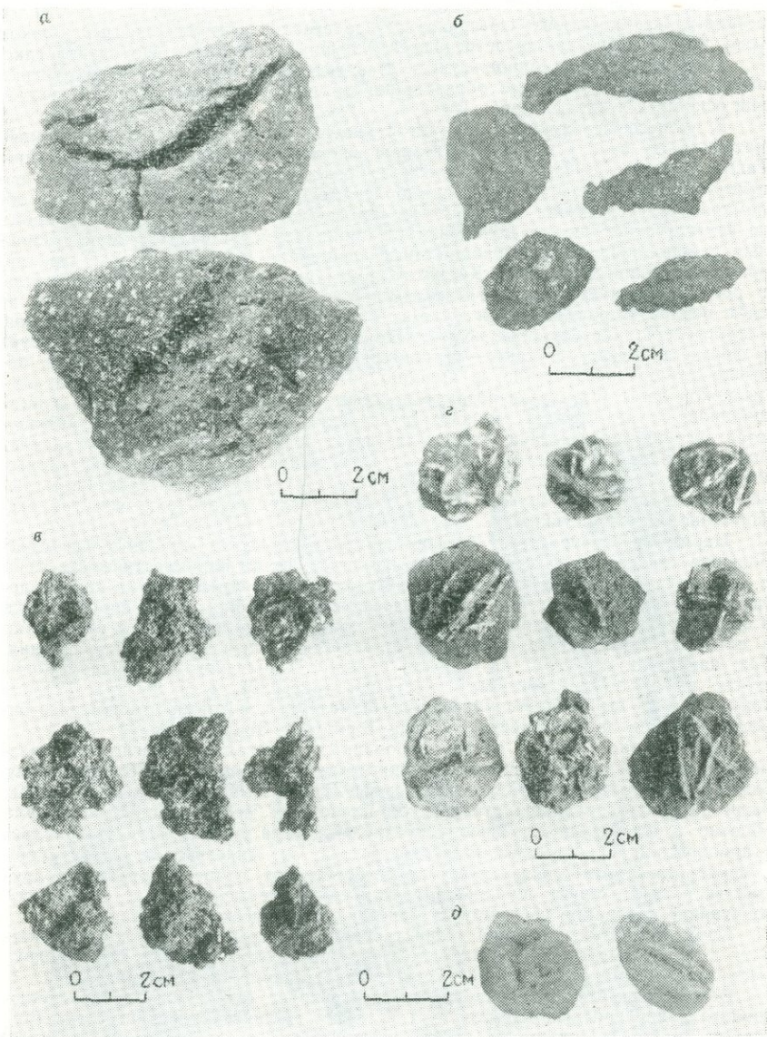
РИС. 29. Пирокластический материал:
