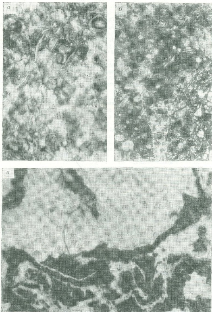
РИС. 26. Гиадокластиты:
