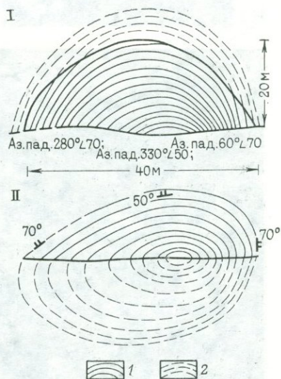
РИС. 52. Купол луковичного строения у с. Оноковцы в Закарпатье:
