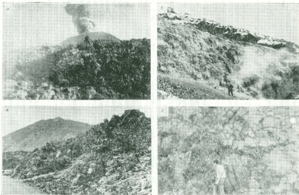
РИС. 24. Брекчиевые лавы:
