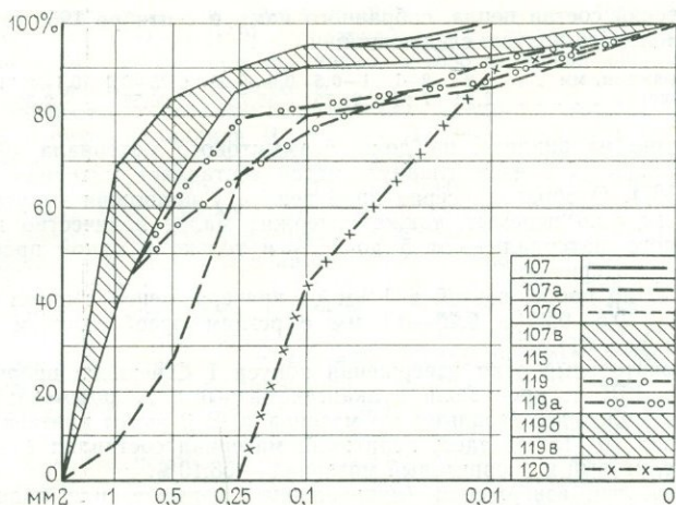
РИС. 62. График гранулометрического состава пеплов вулкана Тятя извержения 1973 г. Проба 107 взята в стороне от оси пеплопада, а проба 120 — в 50 км от центра извержения
