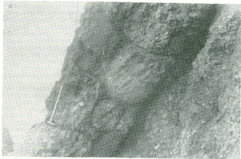
Рис. 49. Подушечные лавы:
