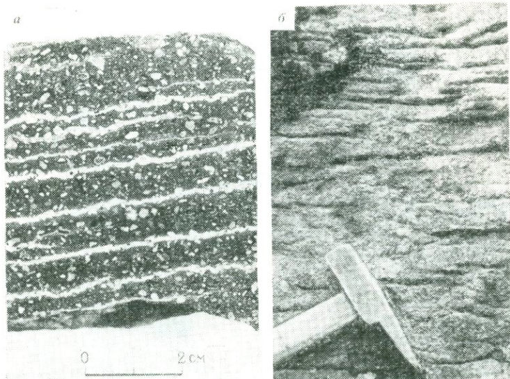
РИС. 5. Плоские поры в андезите: а — в полированном образце; б — в обнажении
