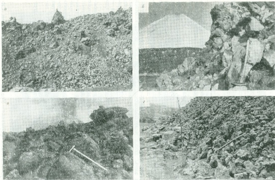
РИС. 25. Лавокластиты:
