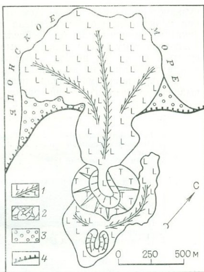
РИС. 37. Заполнение заливов лавовым тефвроидом в течение одного года: 1 — лавовые потоки; 2 — шлаковые конусы; 3 — лавокластитовые тефроида; 4 — первоначальная линия берега
