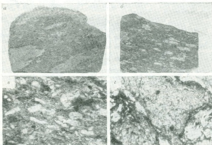
РИС. 68. Псевдоигнимбриды:
