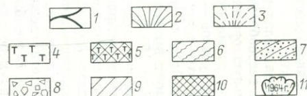
РИС. 54. Разновидности куполов:
