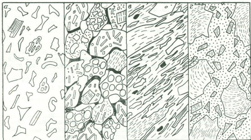
РИС. 22. Структуры, выделяемые по взаимоотношению обломков и цемента: а — структура базального цемента алевритового витрокластического туфа, о. Кунашир; б — структура соприкосновения пор в псаммитовом туфе базальта, Ключевская группа вулканов, Камчатка; в — игнимбритовая структура, Кроноцкий залив, Камчатка; г — вторичнокластолаговая структура, пос. Начики, Камчатка
