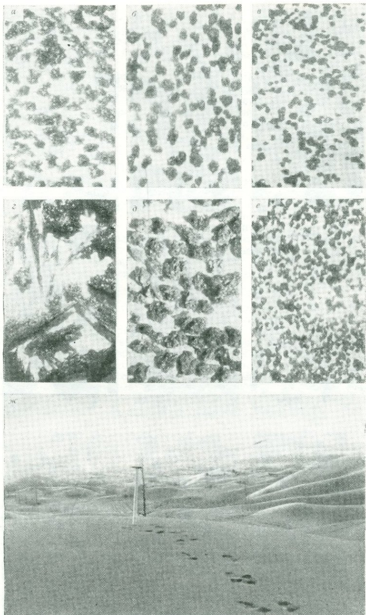
РИС. 31. Вулканические пеплы извержений БТИ и Ключевского, в мм: а — БТИ, 1975 г. (2,0—1,0); б — то же (1,0—0,5); в — то же (0,5—0,25); г — БТИ, 1976 г.; д — Ключевского, 1978 г. (1,0—0,5); е — то же (0,5—0,25) (кол- лекция И. Т. Кирсанова); ж — покров алевропелитового пепла БТИ, выпав- шего 9 августа 1975 г.
