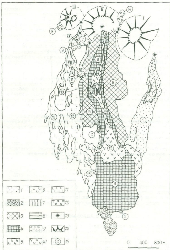
РИС. 43. Лавовые потоки БТТИ, 1975 г. (составил Ю. В. Ванде-Кирков)
