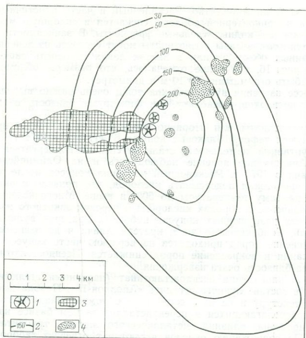
РИС. 61. Распределение мощностей пирокластики Северного прорыва БТТИ, 1975 г. (составил В. А. Будников): 1 — шлаковые конусы; 2 — изогипсы мощностей пирокластики; 3 — лавовые потоки базальта; 4 — шлаковые конусы более ранних извержений.
