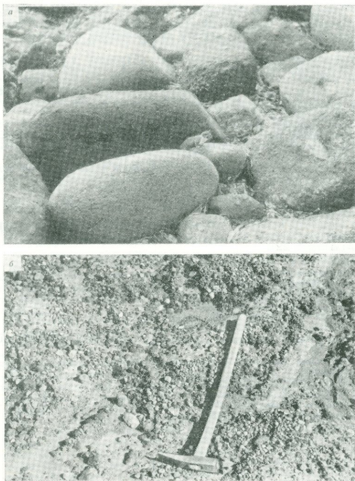
РИС. 38. Вулканотерригенные породы:
