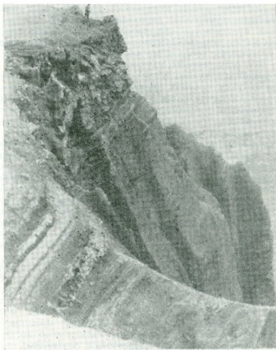
РИС. 60. Слоистая тефра у кратера конуса Такетоми вулкана Алаид с падением в сторону кратера
