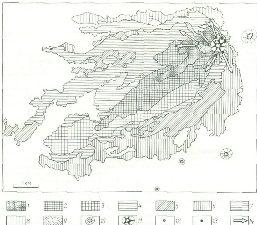
РИС. 39. Лавовые потоки Южного прорыва БТТИ, 1975—1976 гг.
