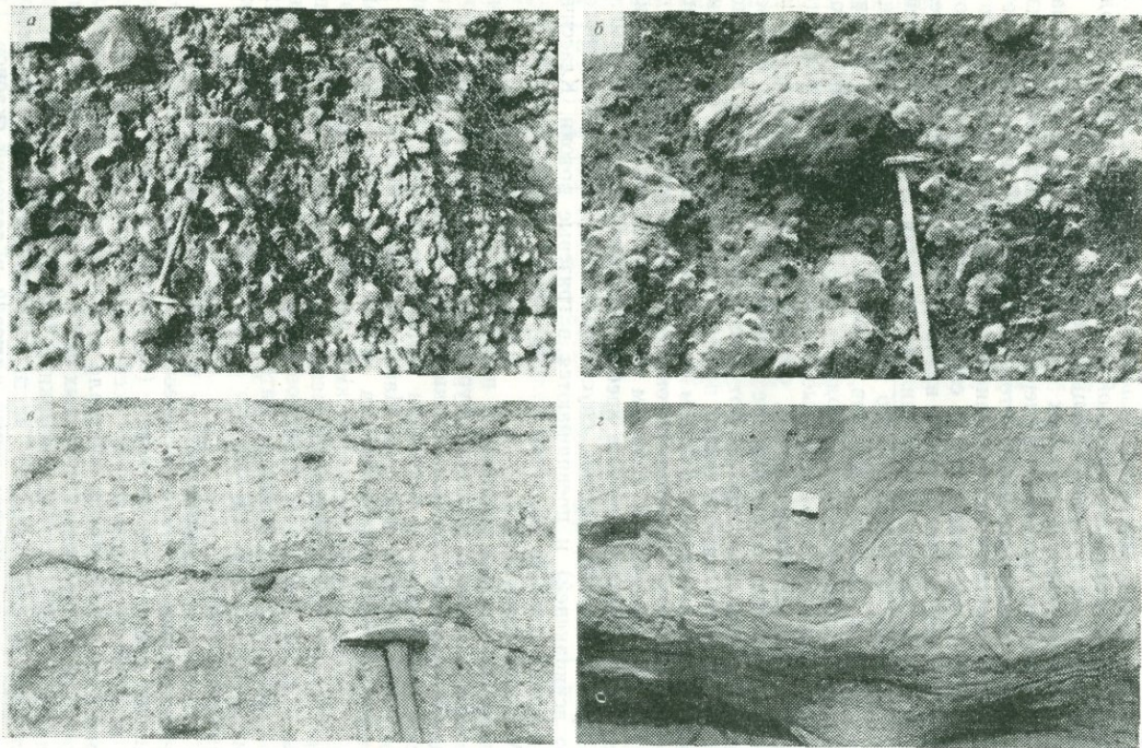
РИС. 69. Отложения грязевых потоков:
