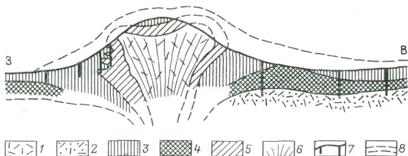
РИС. 3. Строение купола Ардо на окраине г. Бёрегово:
