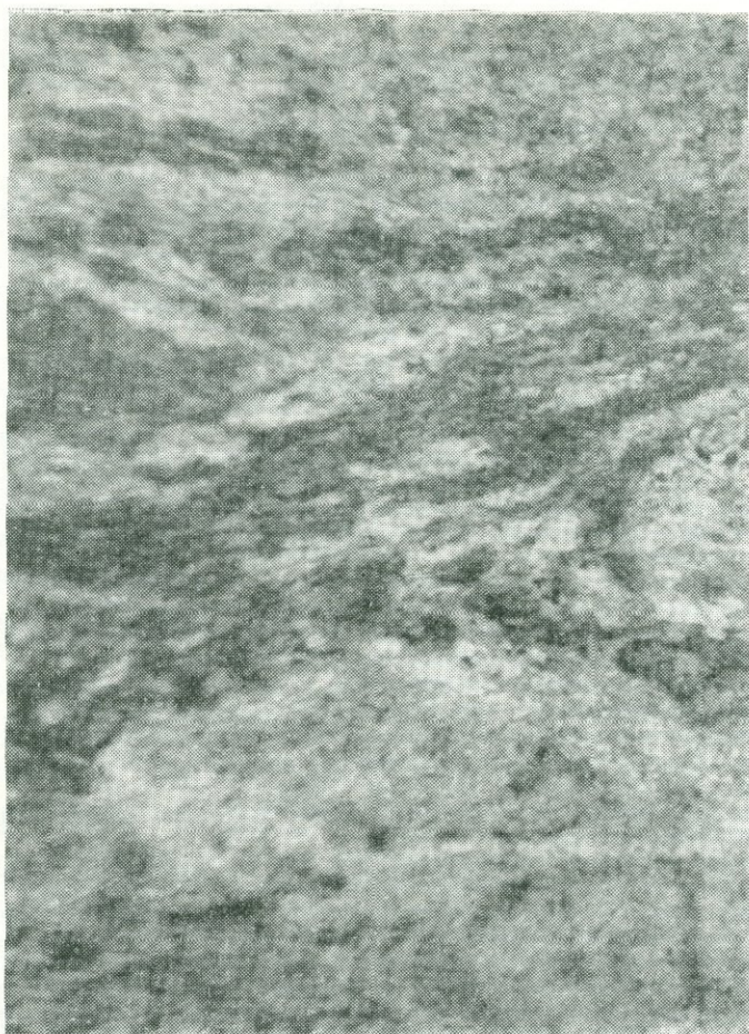
РИС. 48. Игниспумит под микроскопом. Южный Казахстан ( \times 20 )
