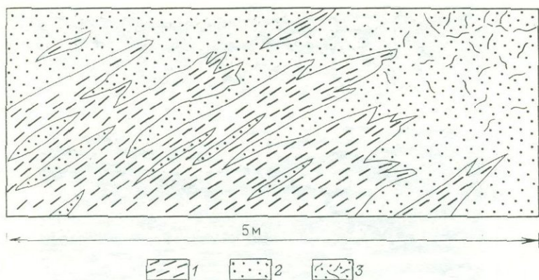
РИС. 45. Переход обсидиана в пемзу: 1 — обсидиан; 2 — пемза; 3 — трещиноватая пемза
