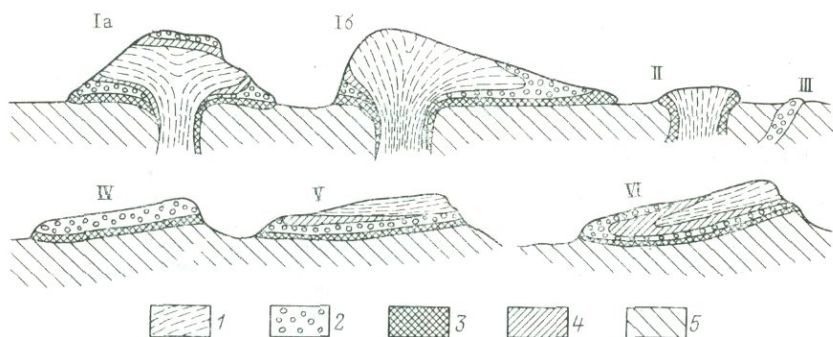
РИС. 2. Формы залегания кислых вулканических стекол:
