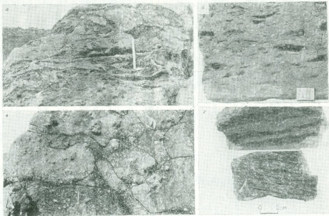
РИС. 15. Текстуры вулканитов:
