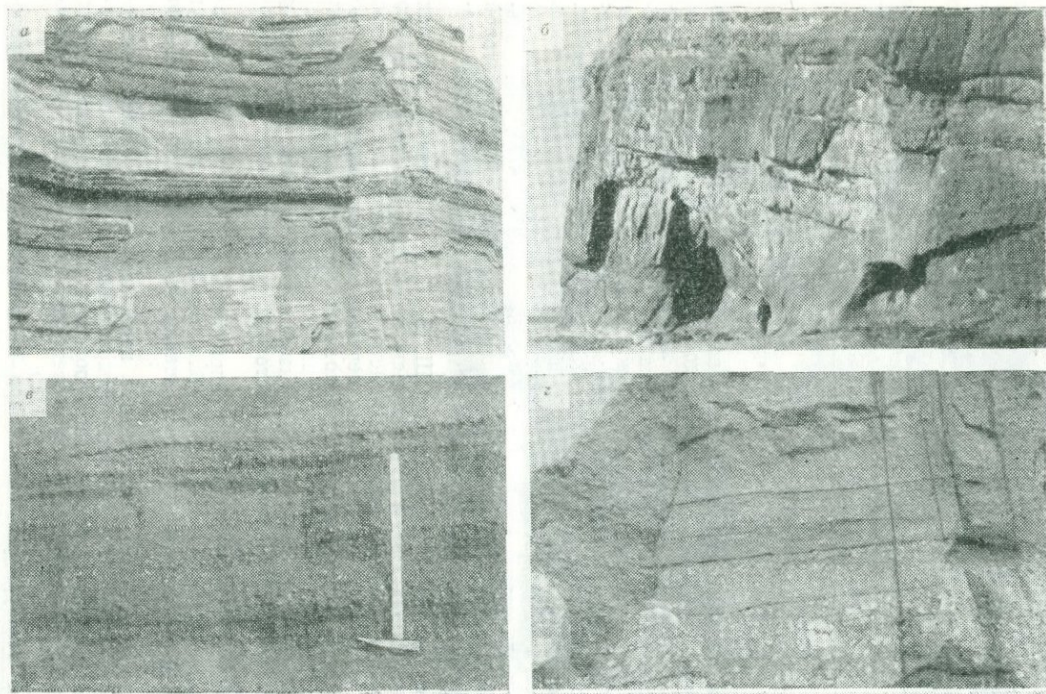
РИС. 19. Слоистые текстуры:
