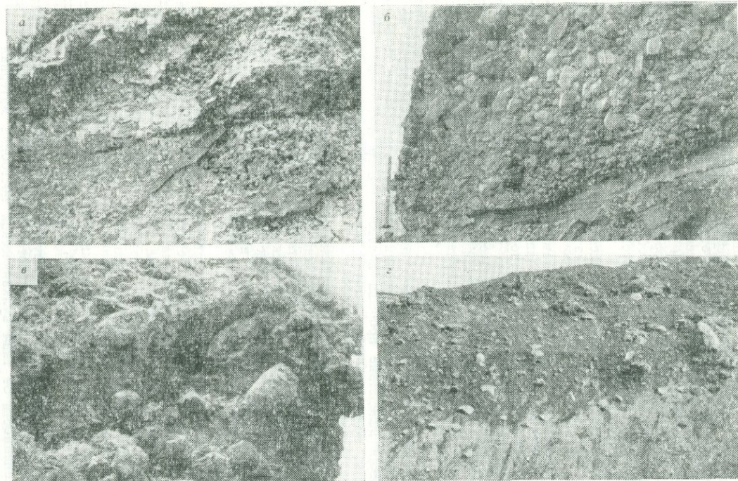
РИС. 34. Грубообломочные туфы:
