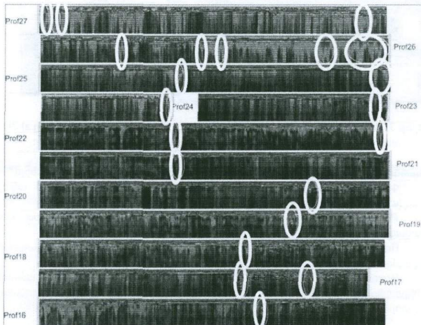
Նկար 2. Երկրորդ տեղամասի գեոռադարային 2D հանույթի պրոֆիլների անոմալիաների գրաֆիկ (անոմալիաները նշված են ռոշկաձև):
