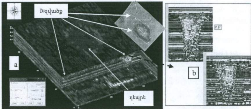
Նկար 3. Երկրորդ տեղամասի գեոռադարային 3D հանույթի մեկնաբանումը a) 3D հանույթի մշակումը b) 3D և 2D հանույթների տվյալների համադրումը:
