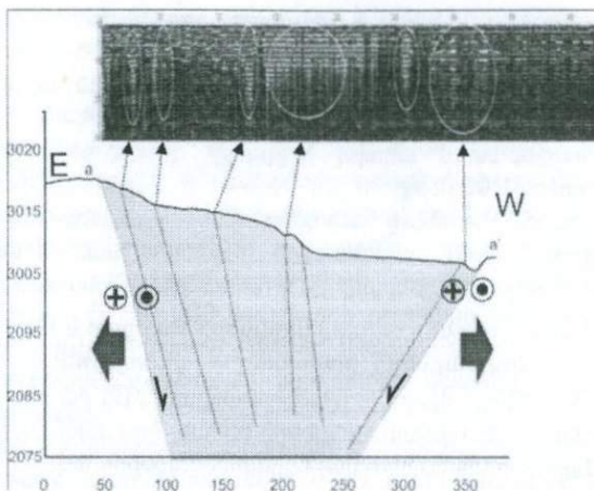
Նկար 4. aa' գեոմորֆոլոգիական պրոֆիլի խախտումները և գեոռադարային հանույթի անոմալիաները:
