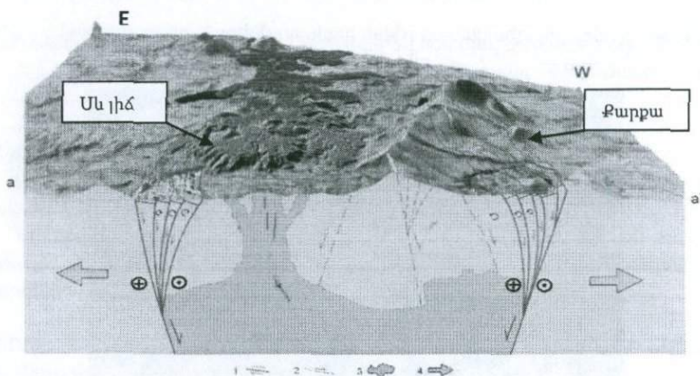
Նկար 6. Փամբակ-Սևան –Սյունիք ակտիվ խզվածքի Քարքար և Սև լիճ տեղամասերի 3D տեկտոնական մոդել 1. Ակտիվ խզվածքներ 2. ենթադրյալ ակտիվ խզվածքներ 3. մագմատիկ օջախ 4. տարածաշրջանային ընդարձակման ուղղությունը:
