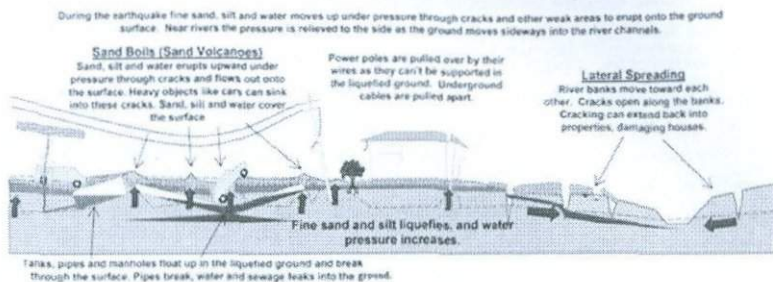
Рисунок 1. Феномен разжижения грунта и его последствия
