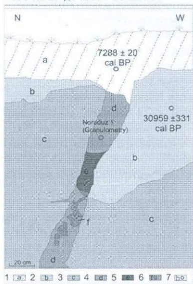
Рисунок 5. Разжижение грунта на окраине села Нурадус. 1. а - слой современной почвы; 2. b - слой вулканической тефры, перемешанные с озерными отложениями Севана прибрежной фации; 3. c - слой вулканической тефры; 4. d - крупнозернистая темная вулканическая тефра; 5. e - черная слоистая мелкозернистая вулканическая тефра; 6. f - обломки песчанника; 7. - места взятия образцов для анализов C14 и гранулометрии.
