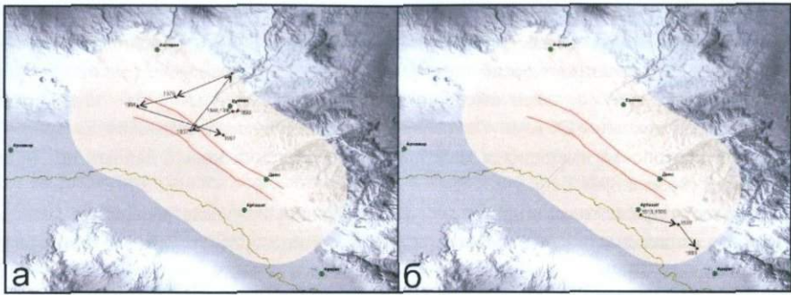
Рис.7. Пространственное расположение и хронологическая последовательность наиболее сильных землетрясений ( M \geq 3,7 ), происшедших: а - в Паракар-Ереванской подзоне до 2017г.; б - в Арташат-Вединской подзоне до 2017г.
