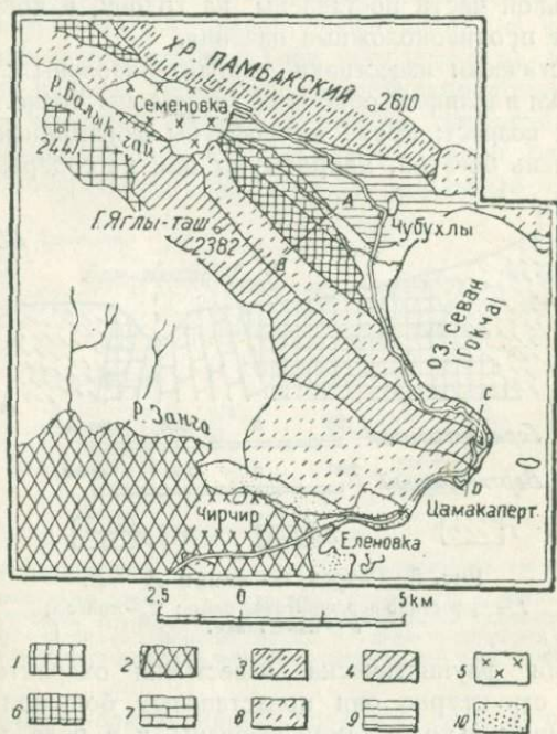
Рис. 4. Геологическая карта района Чубухлы — Еленовка.
