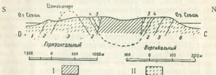
Рис. 6. Разрез по линии С—D.
