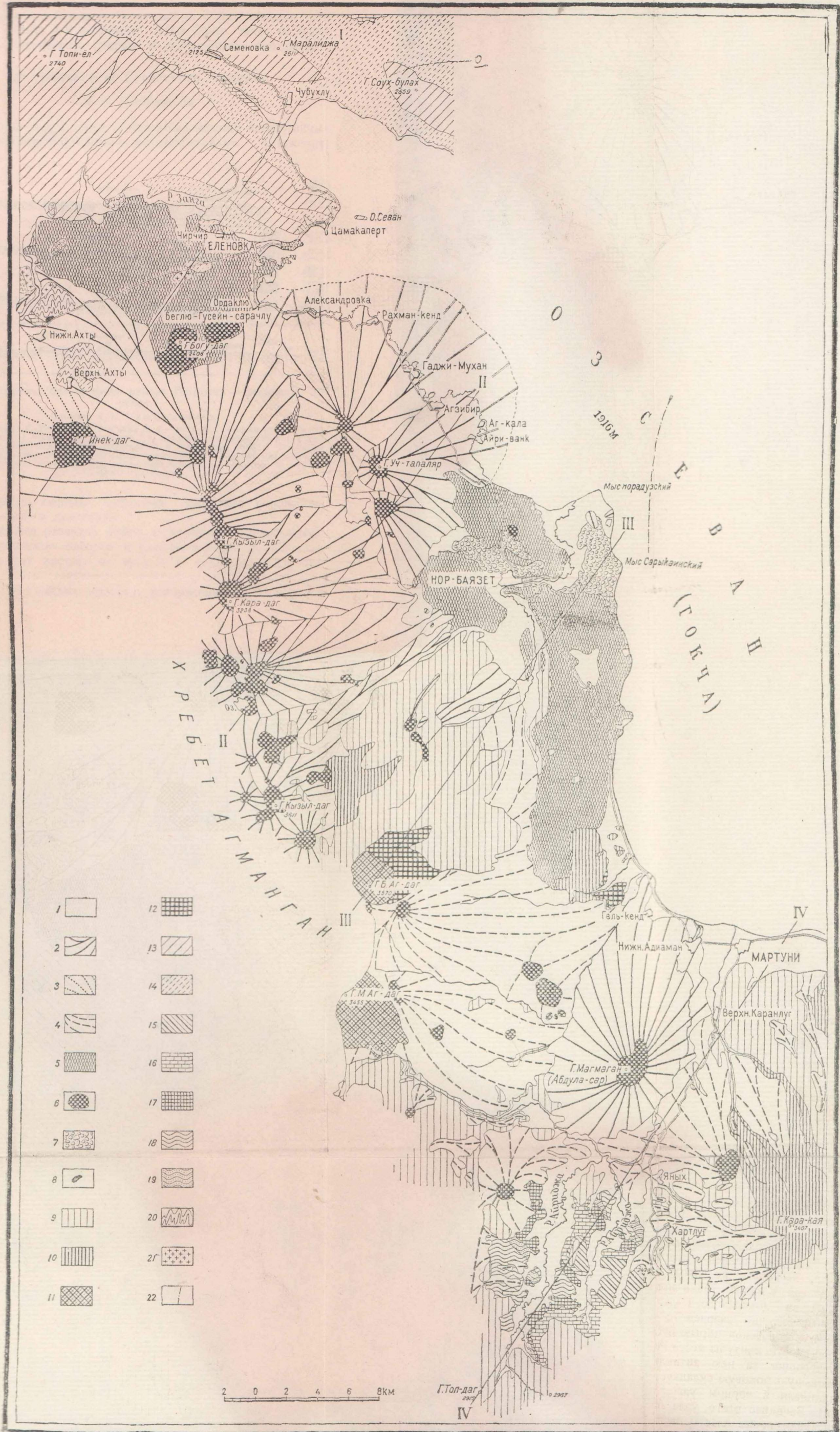
Рис. 7. Геологическая карта западной части бассейна оз. Севан (Гокча). Составил К. Н. Паффенгольц.
