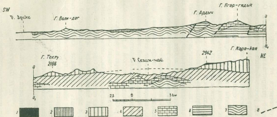
Рис. 13. Геологический профиль района Селимский перевал — Улия-Норашен.
