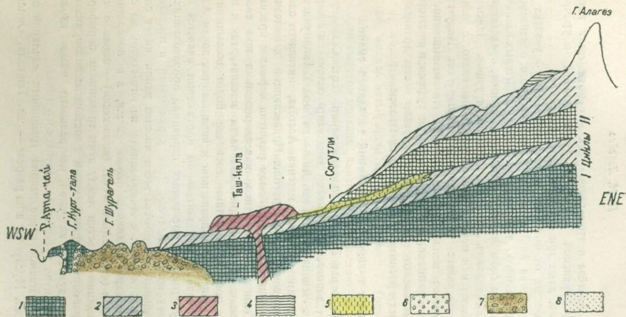
Рис. 17. Схематический геологический разрез горы Алагёз.
