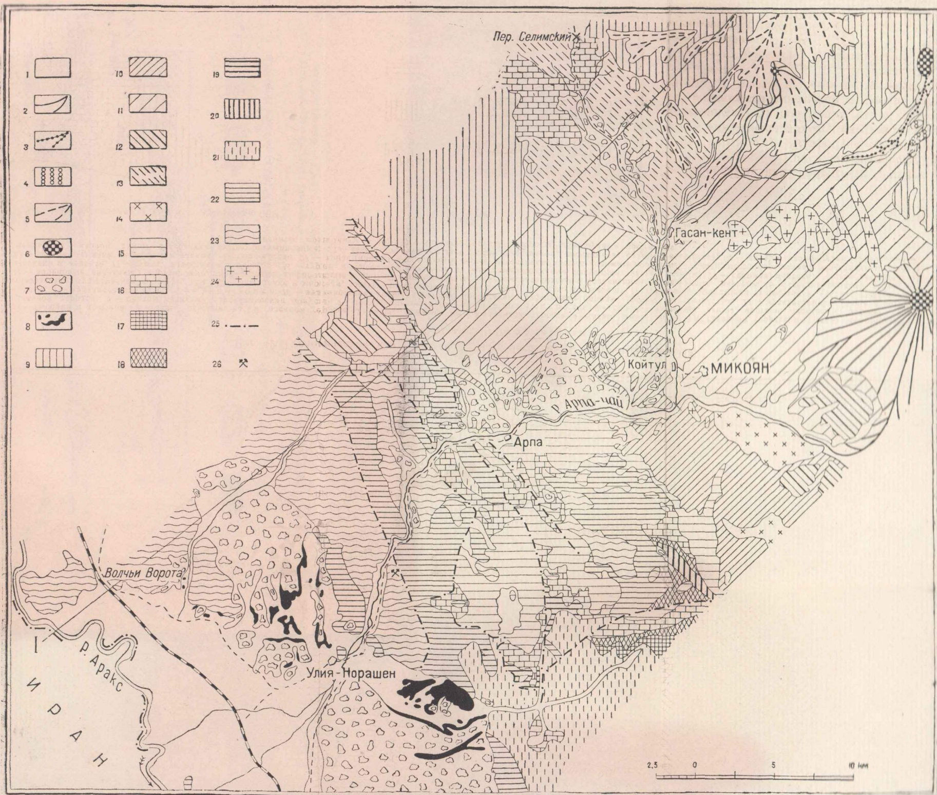
Рис. 12. Геологическая карта западной части бассейна р. Восточный Арпа-чай.
