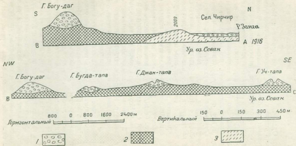
Рис. 11. Геологические разрезы по линиям А—В и В—С. 1 — шлаги; 2 — андезито-базальты; 3 — туфогенно-порфиритовая свита.
