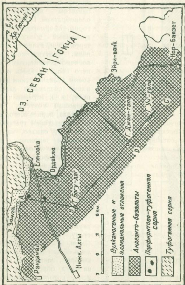
Рис. 9. Геологическая карта района сел. Еленовка — г. Нор-Баязет Составил С. Кузнецов.
