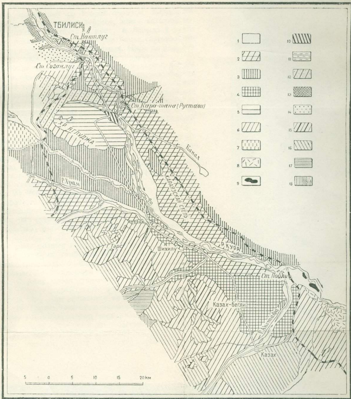
Рис. 1. Геологическая карта района Тбилиси — Казах.
