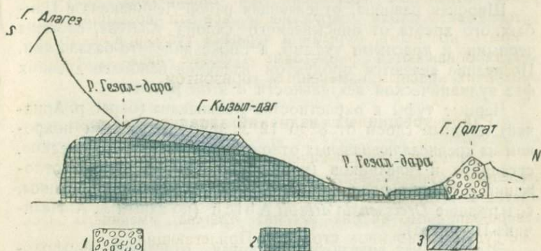
Рис. 18. Схематический геологический разрез северного склона Алагёза.
