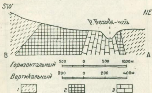
Рис. 5. Разрез по линии A—B .
